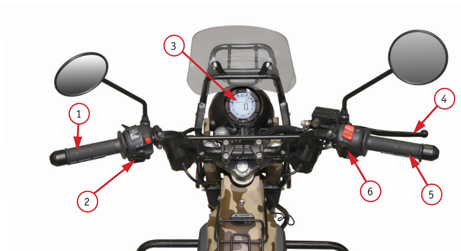
Фото 2.1. Вид руля и органов управления мотоцикла: 1 – левая рулевая рукоятка; 2 – левый комбинированный переключатель; 3 – приборная панель; 4 – ручка переднего тормоза; 5 – рукоятка газа (акселератор); 6 – правый комбинированный переключатель
