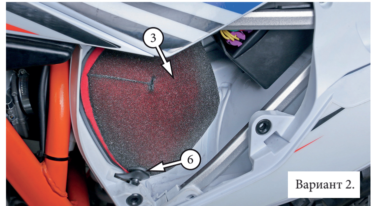
Фото 5.7. Варианты исполнения воздушных фильтров
