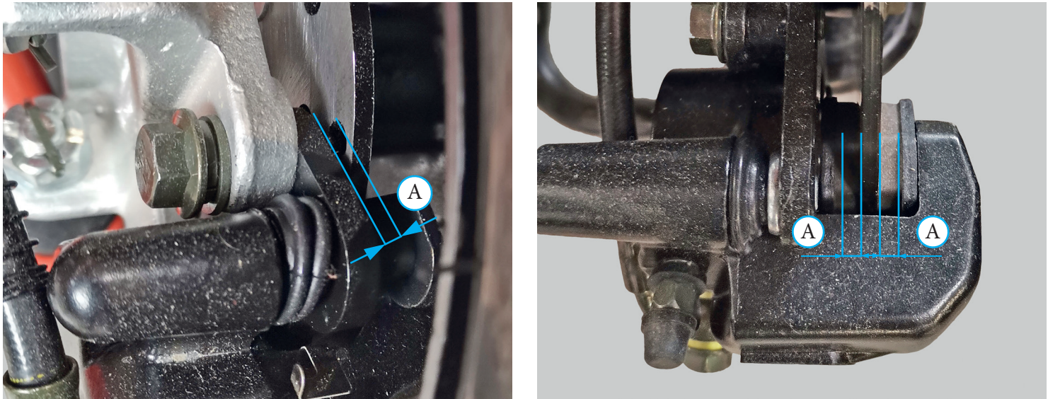
Фото 5.11. Контроль тормозных колодок
