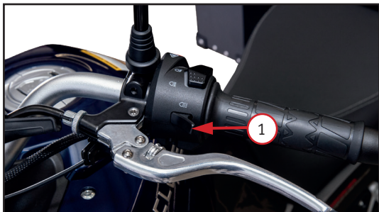
Фото 2.3. Левый комбинированный переключатель (вид спереди): 1 – кнопка включения дальнего света при обгоне
