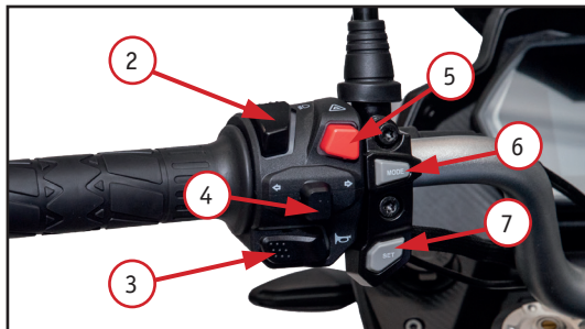
Фото 2.4. Левый комбинированный переключатель: 2 – кнопка переключения режима света фары (дальний свет/ближний свет); 3 – кнопка звукового сигнала; 4 – кнопка указателей поворота; 5 – кнопка включения аварийной сигнализации; 6 – кнопка «MODE»; 7 – кнопка «SET»
