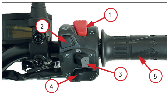
Фото 2.5. Правый комбинированный переключатель: 1 – кнопка включения/отключения питания; 2 – кнопка ABS; 3 – кнопка включения/выключения света фар; 4 – электростартер; 5 – ручка газа (акселератора)
