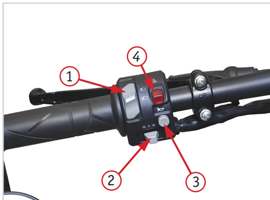
Фото 2.4 Левый комбинированный переключатель: 1 – переключатель режима света фары (дальний свет/ ближний свет); 2 – клавиша указателей поворота; 3 – кнопка звукового сигнала; 4 – кнопка аварийной сигнализации; 5 – кнопка включения дальнего света при обгоне
