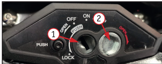
Фото 2.7. Комбинированный замок для модели ZT125-Z2:1 – замочная скважина; 2 – гнездо поворотной защиты.
