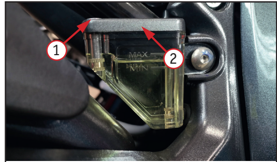
4.9.2. Бачок тормозной жидкости задних тормозов: 1 – винты крепления крышки бачка; 2 – крышка бачка.
