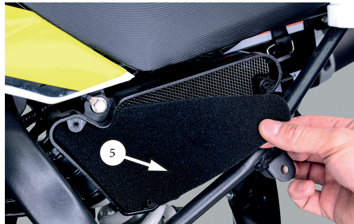
Фото 5.7. Обслуживание воздушного фильтра закрытого типа
