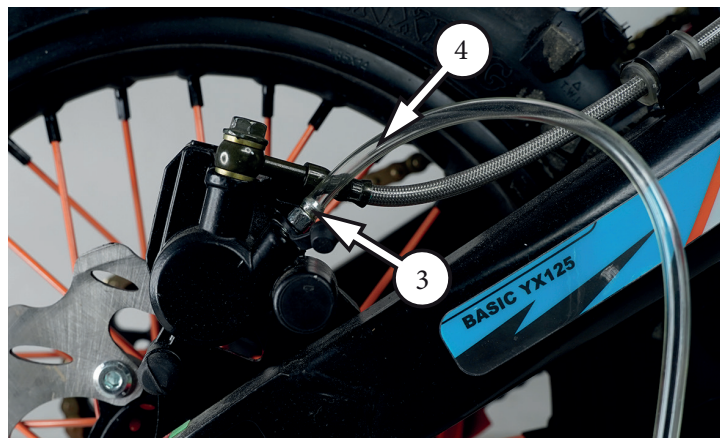
Фото 5.20. Прокачка тормозных контуров
