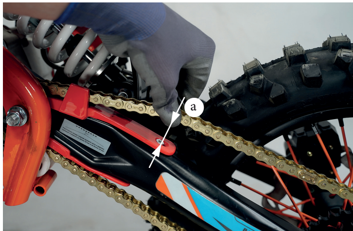
Фото 5.23. Замер провисания цепи
