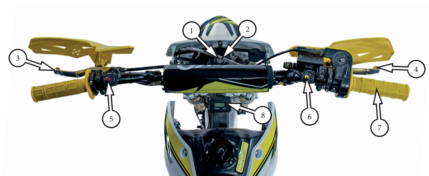
Фото 2.3 Приборы и органы управления: 1 – замок зажигания; 2 – вкл./выкл. фары (не на всех моделях); 3 – рычаг сцепления; 4 – рычаг переднего тормоза; 5 – кнопка выключения двигателя; 6 – кнопка стартера; 7 – рукоятка акселератора; 8 – приборная панель/счетчик моточасов
