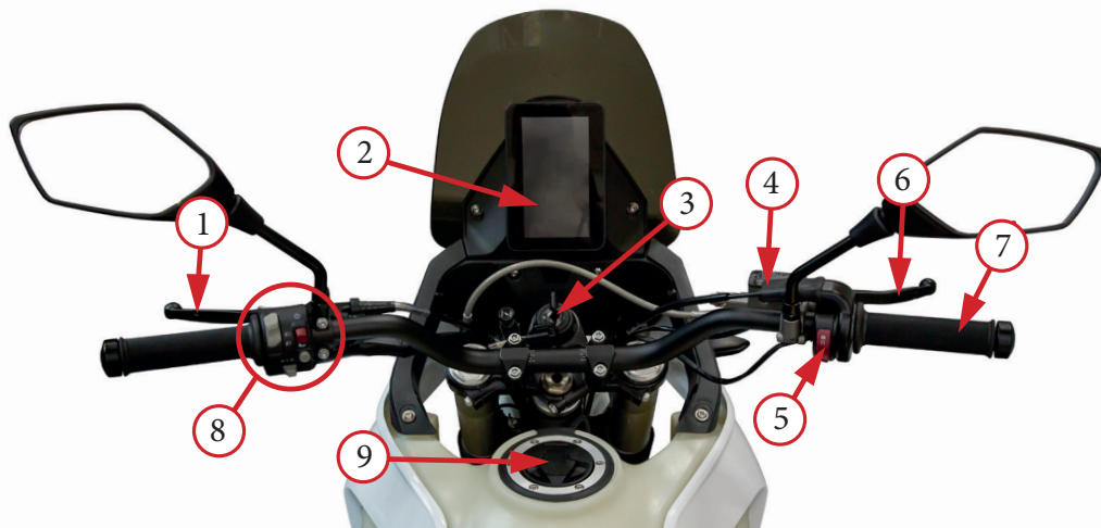
Фото 2.4 Органы управления на примере мотоцикла GR S3 RALLY: 1 – рычаг сцепления; 2 – приборная панель; 3 – замок зажигания; 4 – бачок тормозной жидкости передних тормозов; 5 – кнопка включения/отключения питания двигателя и электростартера; 6 – рычаг переднего тормоза; 7 – ручка акселератора (газа); 8 – левый блок переключателей; 9 – крышка бензобака; 10 – кнопка мигания дальним светом; 11 – кнопка включения света фар; 12 – кнопка переключения режима фары (дальний/ближний свет); 13 – переключатель указания поворотов; 14 – кнопка звукового сигнала
