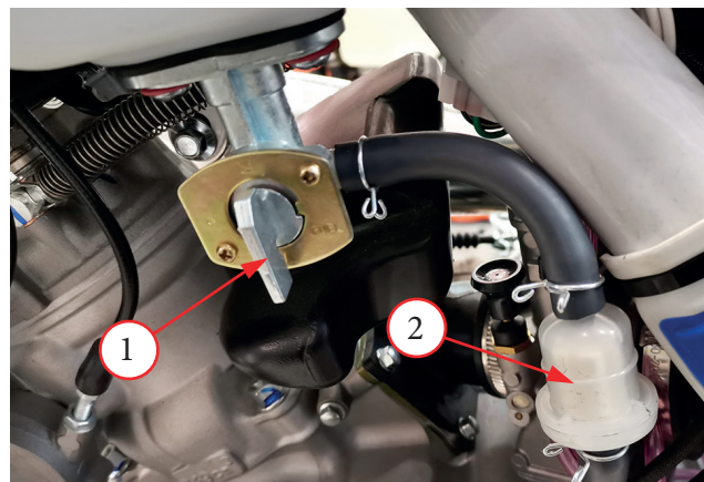
Фото 3.2. Место установки: 1 - топливный кран; 2 - топливный фильтр
