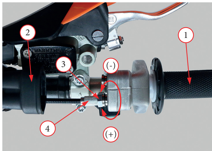
Фото 5.8. Регулировка свободного хода рукоятки акселератора
