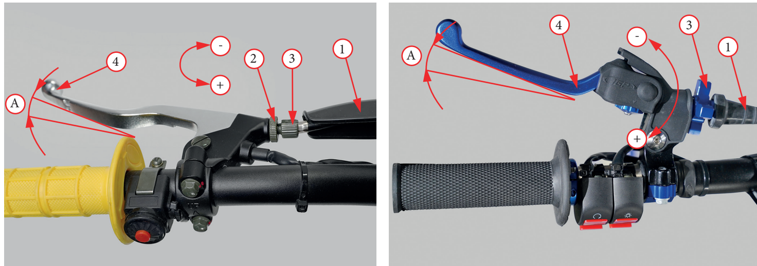
Фото 5.10. Регулировка свободного хода рычага сцепления (варианты исполнения)
