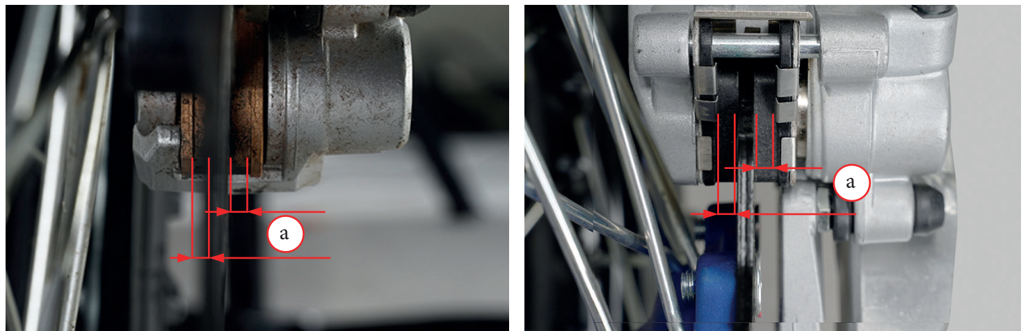
Фото 5.18. Контроль тормозных колодок
