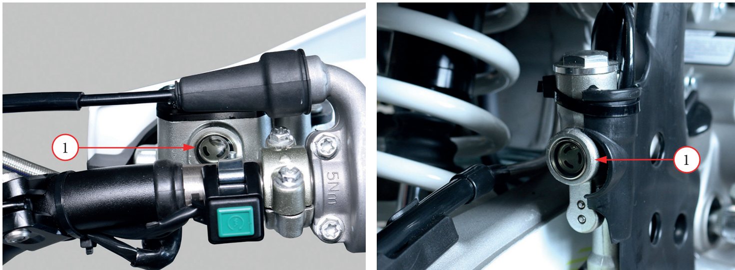
Фото 5.17. Контроль и долив тормозной жидкости
