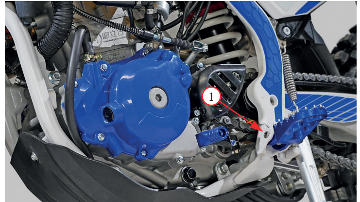
Фото 5.24. Слайдер-успокоитель – 1 (расположен за рамой)
