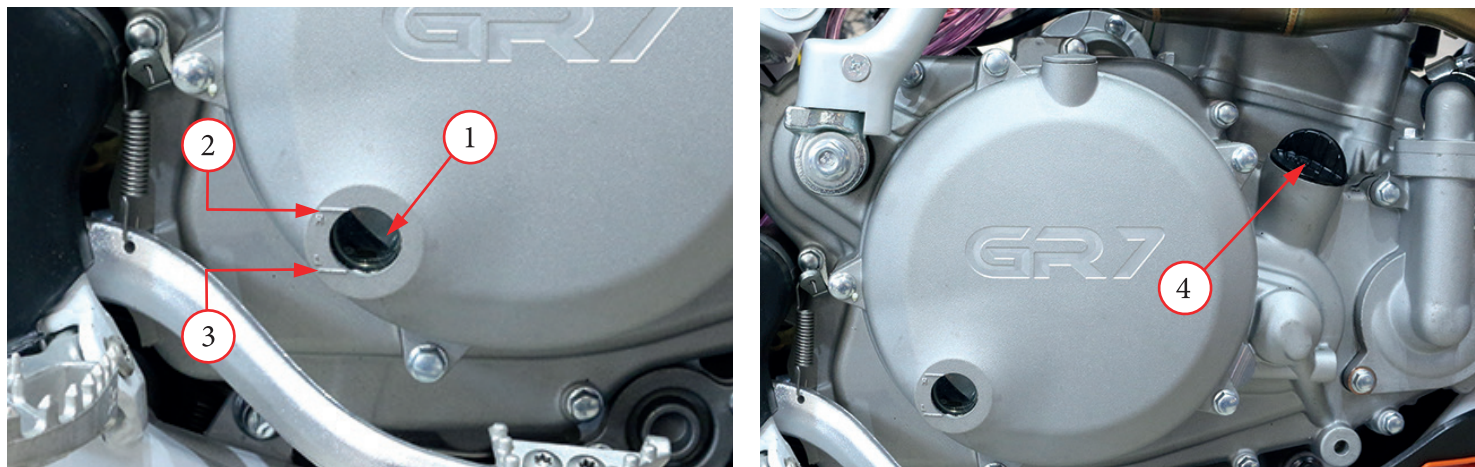
Фото 5.3. Варианты исполнения смотрового окна и крышки горловины двигателей. 1 - смотровое окно с указателями уровня (максимум - «2» и минимум - «3»); 4 – крышка маслозаливной горловины
