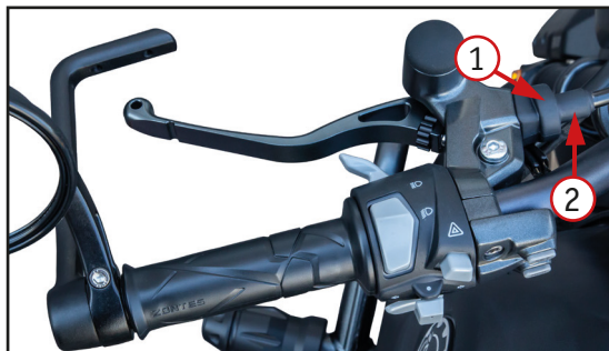
Фото 3.4. Регулировка рычага сцепления на руле (под колпаком): 1 – стопорная гайка; 2 – регулировочная гайка
