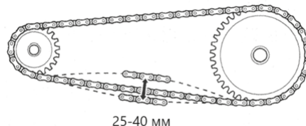
Рисунок 4. Натяжение цепи
