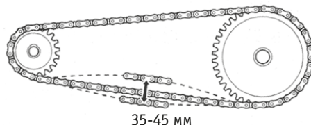
Рисунок 3. Натяжение цепи
