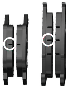
Фото 4.10. Контрольные канавки тормозных колодок
