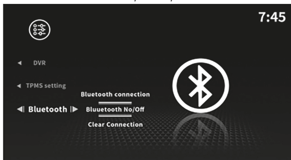
Фото 2.8.8 Настройка Bluetooth
