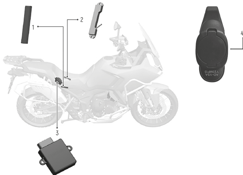
Фото 2.6. Система бесключевого доступа: 1 – приемно-передающая антенна; 2 – индуктивная антенна; 3 – блок управления РКЕ; 4 – активный ключ
