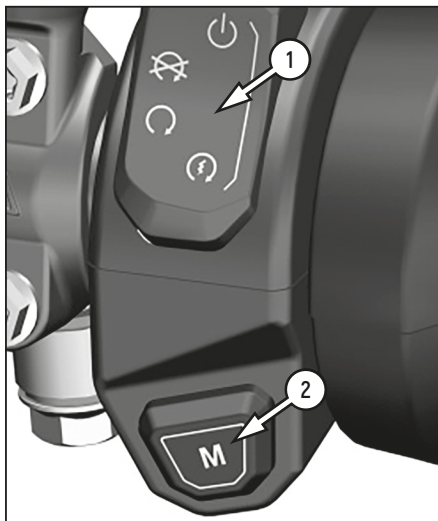
Фото 2.5 Правый блок переключателей:
