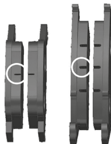
Фото 4.11. Канавки износа тормозных колодок
