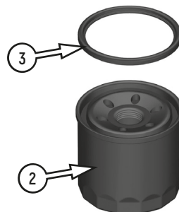
Фото 4.7. Замена масляного фильтра: 1 – защита фильтра; 2 – масляный фильтр; 3 – уплотнительное кольцо
