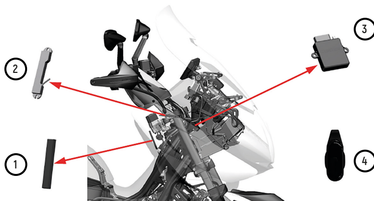
Фото 2.6. Система бесключевого доступа: 1 – приемо-передающая антенна; 2 – индуктивная антенна; 3 – блок РКЕ; 4 – активный ключ
