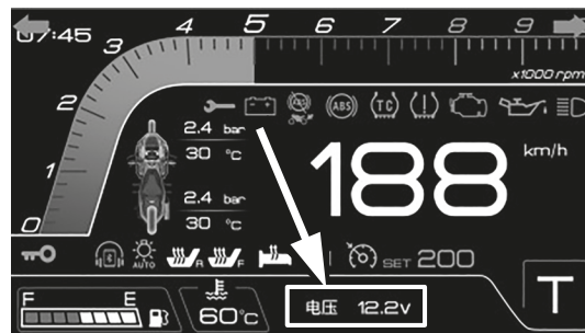
Фото 2.8.2. Индикатор напряжения
