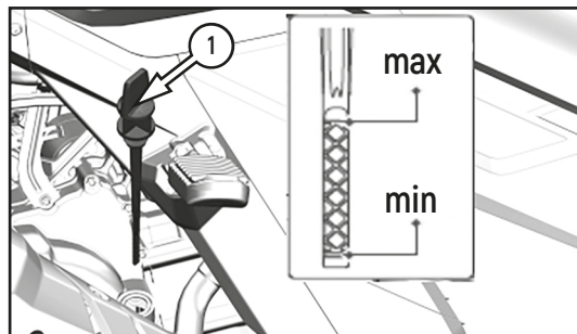
Фото 2.20. Проверка масла по щупу 1
