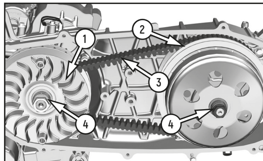
Фото 4.10. Передаточный механизм: 1 – ведущий шкив; 2 – ведомый шкив; 3 – клиновой ремень; 4 – места смазки
