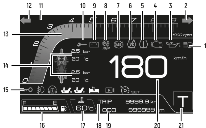
Фото 2.8. Приборная панель: 1 - индикатор дальнего света; 2 - указатель поворота направо; 3 - индикатор низкого давления моторного масла; 4 - индикатор неисправности двигателя; 5 - индикатор давления в шинах; 6 - индикатор системы курсовой устойчивости (TCS); 7 - индикатор системы ABS; 8 - задний индикатор отключения ABS (для модели 368E-G); 9 - индикатор низкого напряжения батареи; 10 - индикатор необходимости проведения ТО; 11 - место индикатора часов (для модели 368T-D/M); 12 - указатель левого поворота; 13 - тахометр "x1000об/мин"; 14 - индикация о низком давлении в шинах и температуре; 15 - индикатор идентификации ключа; 16 - указатель уровня топлива; 17 - температура охлаждающей жидкости; 18 - счетчик текущего пробега TRIP; 19 - счетчик общего пробега ODO; 20 - указатель скорости; 21 - указатель выбранного режима (туристический/спортивный)
