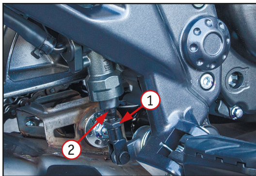
Фото 3.6. Регулировка положения педали заднего тормоза: 1 – стопорная гайка; 2 – шток цилиндра
