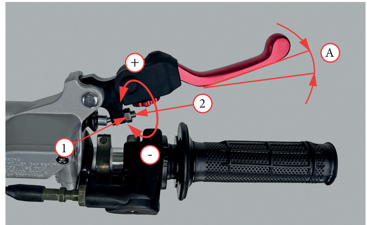
Фото 5.17. Регулировка передних тормозов
