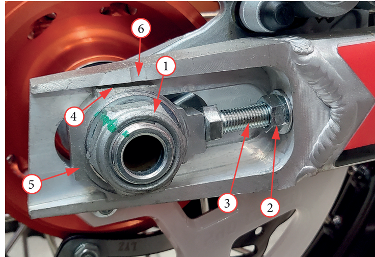
Фото 5.29. Регулировка натяжения цепи
