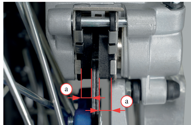
Фото 5.21. Контроль тормозных колодок
