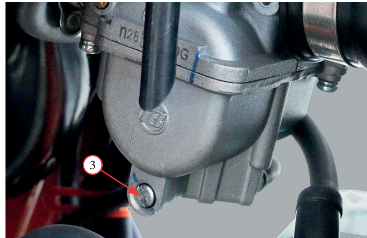
Фото 5.10. Регулировка холостых оборотов
