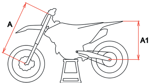
Рисунок 5.25. Замеры на подставке
