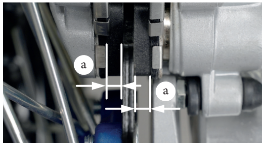
Фото 5.17. Контроль тормозных колодок
