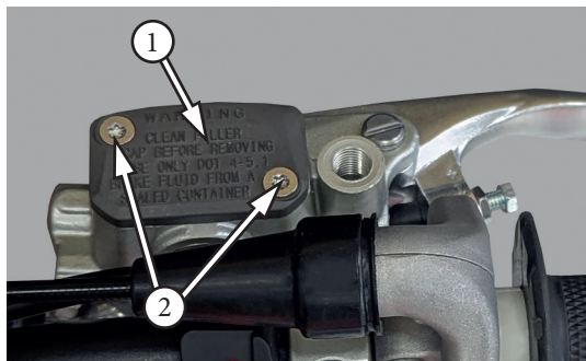
Фото 5.16. Долив тормозной жидкости: 1 – крышка; 2 – винты крепления
