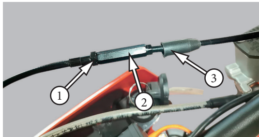
Фото 5.71. Регулировка свободного хода рукоятки акселератора на тросе: 1 – стопорная гайка; 2 – регулятор; 3 – резиновый пыльник
