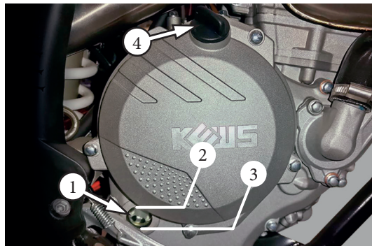
Фото 5.2 Смотровое окно 1 и крышка маслозаливной горловины 4 (вариант): 2 – уровень «максимум», 3 – уровень «минимум»
