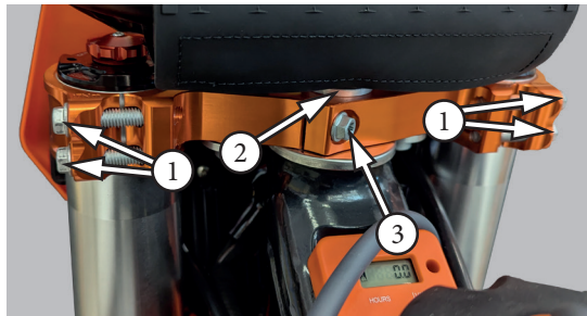
Фото 5.24. Регулировка подшипников рулевой колонки: 1 – болты верхней траверсы; 2 – регулировочный болт (под подушкой); 3 – зажимной болт
