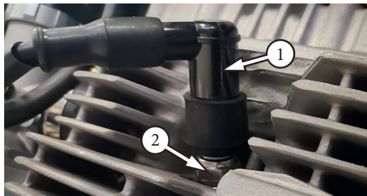
Фото 3.3. Свеча зажигания 2 с колпачком 1
