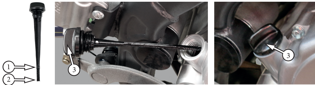
Фото 5.3. Указатель уровня масла в двигателях: 1 – уровень «МАКСИМУМ»; 2 – уровень «МИНИМУМ»; 3 – щуп (крышка горловин)
