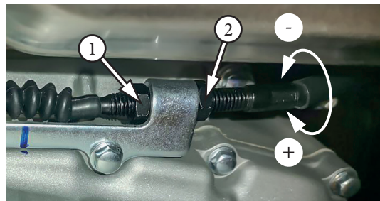
Фото 5.10. Регулировка сцепления на двигателе (вариант): 1 – стопорная гайка; 2 – гайка регулятора
