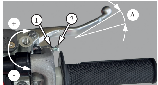
Фото 5.14. Регулировка передних тормозов: 1 – контргайка; 2 – регулятор
