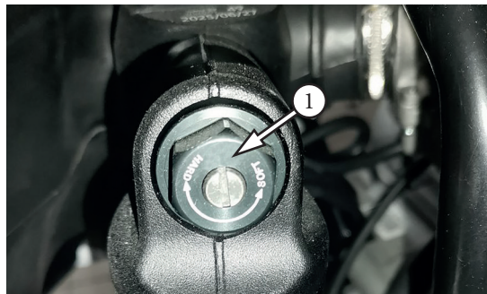
Фото 5.28. Регулятор сжатия – 1 задней подвески
