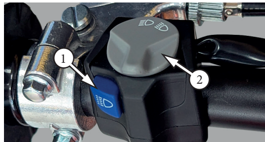
Фото 2.6. Блок переключения фары: 1 – кратковременное включение дальнего света; 2 – переключатель ближнего/дальнего света
