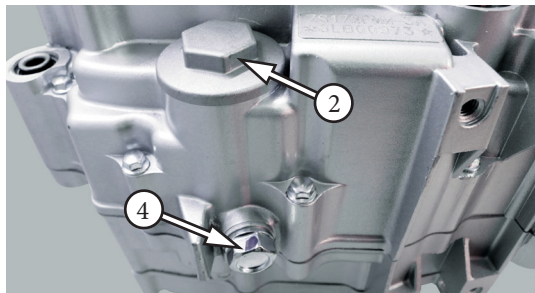
Фото 5.5. Замена масла в двигателях: крышка - 2; фильтр - сетка - 3; сливной болт - 4
