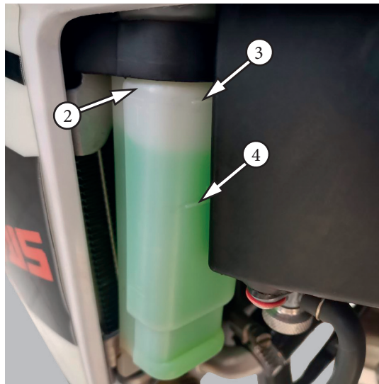
Фото 5.6. Контроль уровня охлаждающей жидкости: 1 – крышка радиатора; 2 – бачек; 3 – уровень «максимум»; 4 – уровень «минимум»
