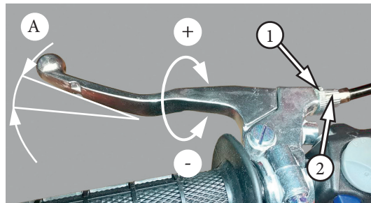
Фото 5.9. Регулировка свободного хода рычага сцепления (вариант): 1 – стопорная гайка; 2 – регулятор троса; А – величина свободного хода
