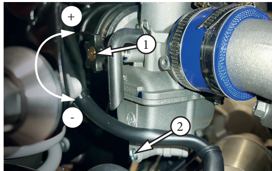
Фото 5.8. Регулировка холостых оборотов (вариант): 1 – винт холостых оборотов; 2 – винт качества
