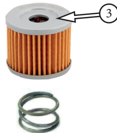
Фото 54. Замена масла в двигателях с масляным фильтром: 1 – крышка маслосаливной горловины; 2 – болты крепления крышки масляного фильтра; 3 – масляный фильтр
