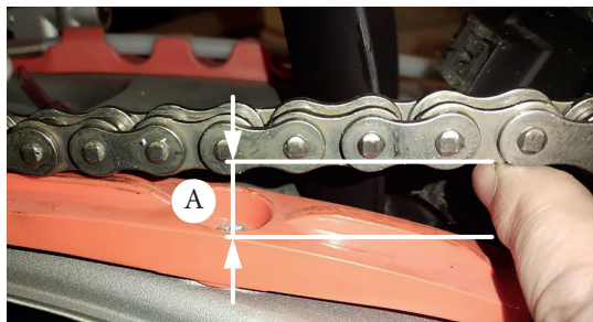
Фото 5.18. Замер провисания цепи
