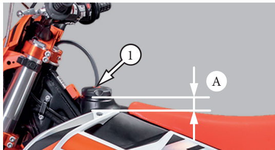
Фото 5.1. Уровень заправки «А» топливного бака
