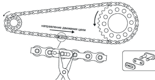
Рисунок 5.22. Установка элементов замка цепи
