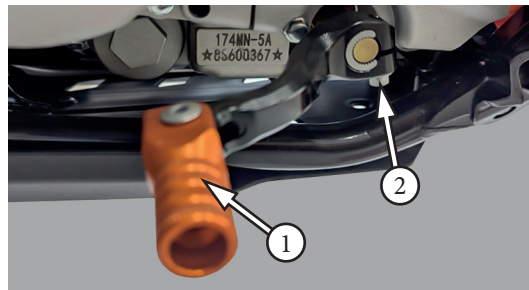
Фото 5.11. Регулировка положения рычага передач: 1 – рычаг передач; 2 – фиксирующий болт
