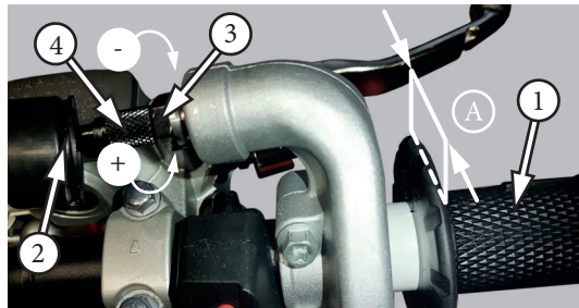
Фото 5.72. Регулировка свободного хода рукоятки акселератора на ручке [вариант]: 1 – ручка акселератора; 2 – резиновый пыльник; 3 – стопорная гайка; 4 – регулятор; A – величина свободного хода
