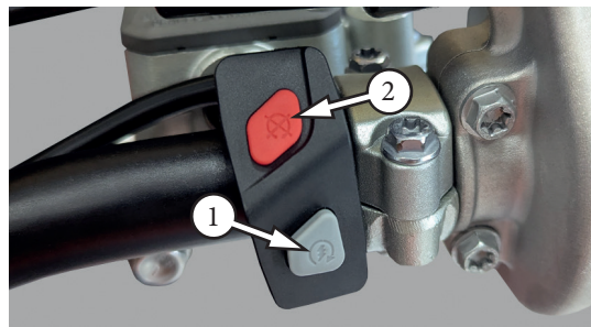
Фото 3.5.2 Кнопки: 1 – запуска двигателя; 2 – остановки двигателя
