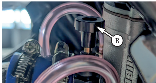
Фото 3.2. Рычаг обогапителя топливной смеси – В
