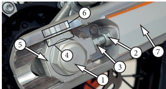
Фото 5.21. Регулировка натяжения цепи
