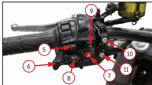
Фото 2.4. Левый комбинированный переключатель: 5 – переключатель поворотников; 6 – кнопка понижения передачи; 7 – кнопка TCS (система стабилизации); 8 – кнопка сигнала (зудок); 9 – кнопка аварийной сигнализации; 10 – кнопка M; 11 – кнопка S
