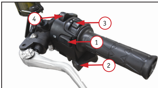
Фото 2.3. Левый комбинированный переключатель (вид спереди): 1 – кнопка включения дальнего света при обгоне; 2 – кнопка повышения передачи, 3 – переключатель режимов КПП; 4 – переключатель дальнего/ближнего света
