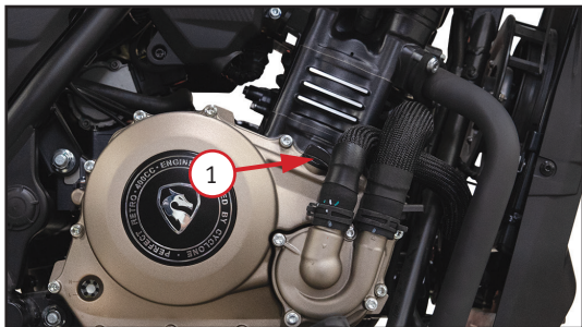
Фото 5.5. Горловина для залива масла 1, болт слива масла 2
