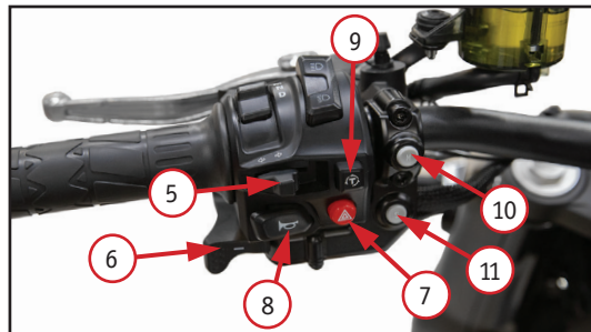
Фото 2.4. Левый комбинированный переключатель: 5 – переключатель поворотников; 6 – кнопка понижения передачи; 7 – кнопка TCS (система стабилизации); 8 – кнопка сигнала (гудок); 9 – кнопка аварийной сигнализации; 10 – кнопка M; 11 – кнопка S
