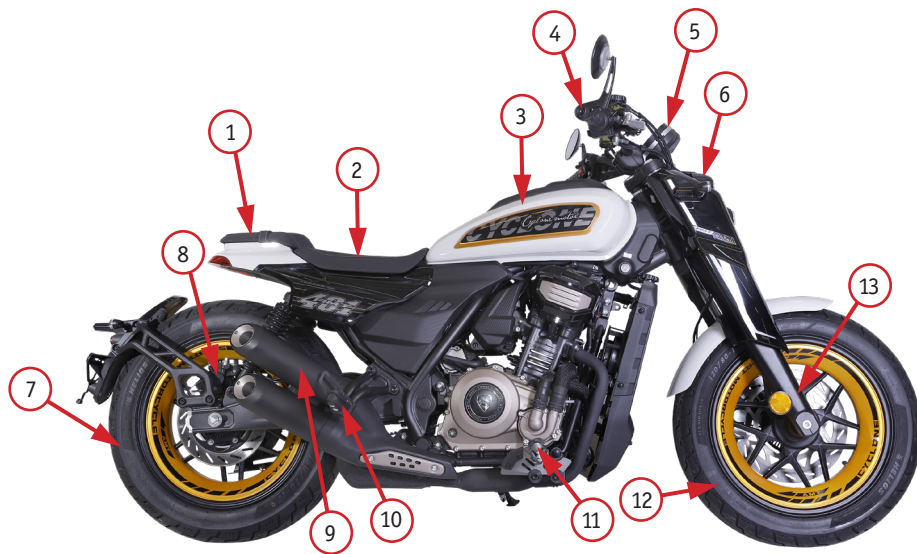
Фото 2.2. Вид мотоцикла: 1 – пассажирское сиденье; 2 – сиденье водителя; 3 – топливный бак; 4 – руль; 5 – приборная панель; 6 – фара; 7 – заднее колесо; 8 – задний тормозной суппорт; 9 – глушитель; 10 – подножка пассажира; 11 – подножка водителя; 12 – переднее колесо; 13 – передний амортизатор
