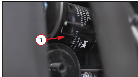
Фото 5.6. Замена масляного фильтра 3
