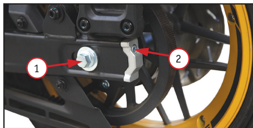
Фото 5.9 Регулировка ремня: 1 – гайка задней оси; 2 – регулировочный болт
