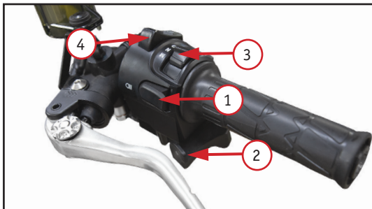
Фото 2.3. Левый комбинированный переключатель (вид спереди): 1 – кнопка включения дальнего света при обгоне; 2 – кнопка повышения передачи, 3 – переключатель режимов КПП; 4 – переключатель дальнего/ближнего света
