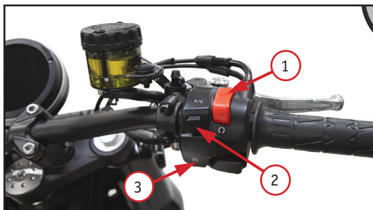
Фото 2.5. Правый комбинированный переключатель: 1 – кнопка включения/отключения питания; 2 – кнопка выбора режима мощности; 3 – электростартер
