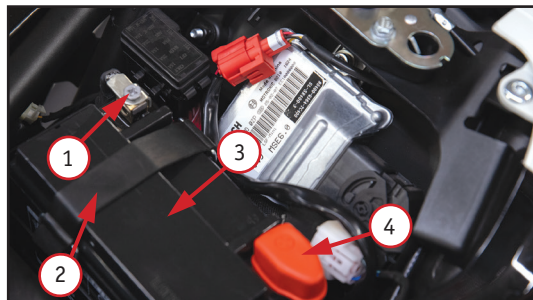
Фото 4. Аккумуляторный отсек и блок предохранителей: 1 – клемма «минус»; 2 – крепеж аккумуляторной батареи (АКБ); 3 – аккумуляторная батарея; 4 – клемма «плюс»
