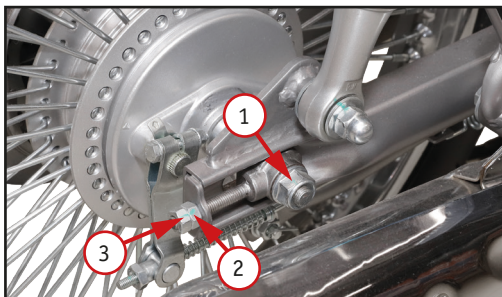
Фото 5.8. Регулировка натяжения цепи: 1 – гайка оси; 2 – регулировочный болт; 3 – стопорная гайка
