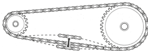
Рисунок 2. Натяжение цепи
