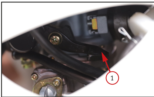
Фото 3.2. Рычаг воздушной заслонки (обогащения топливной смеси) – 1
