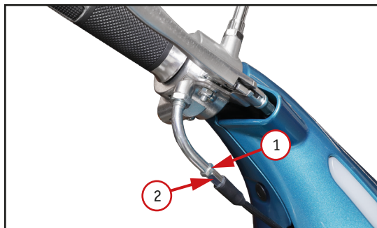
Фото 5.4. Регулировка троса газа: 1 – стопорная гайка; 2 – регулировочная гайка
