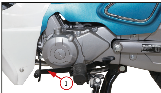
Фото 2.9. Рычаг переключения передач – 1
