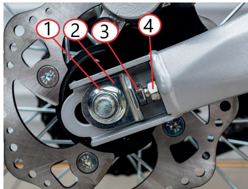
Фото 5.13. Регулировка натяжения цепи: 1 – гайка; 2 – натяжитель; 3 – регулировочный болт; 4 – контргайка
