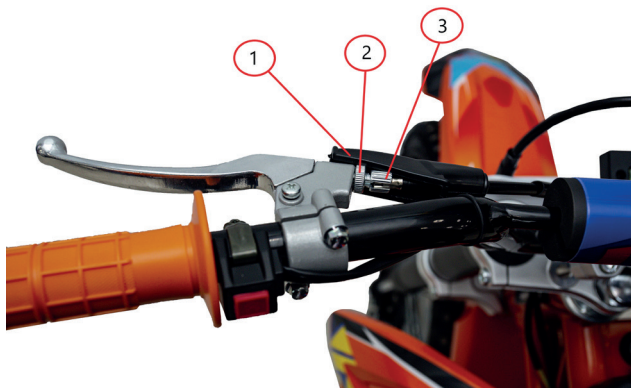
Фото 5.7. Регулировка свободного хода рычага сцепления: пылезащитный колпак 1; стопорная гайка 2; регулятор 3
