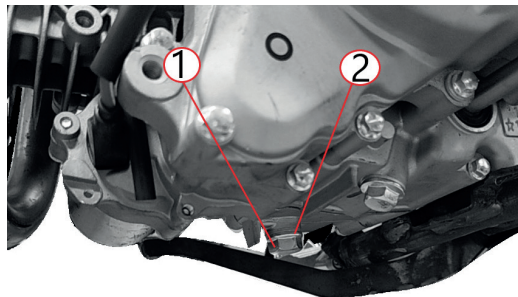
Фото 5.3. Замена масла: сливной болт 1; шайба 2
