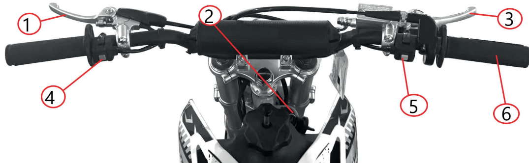
Фото 2.3. Приборы и органы управления: 1 – рычаг сцепления; 2 – ключ с замком зажигания; 3 – рычаг переднего тормоза; 4– кнопка выключения двигателя; 5 – кнопка стартера; 6 – рукоятка акселератора(газа)
