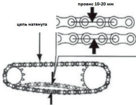
Рисунок 2. Замер провисания цепи
