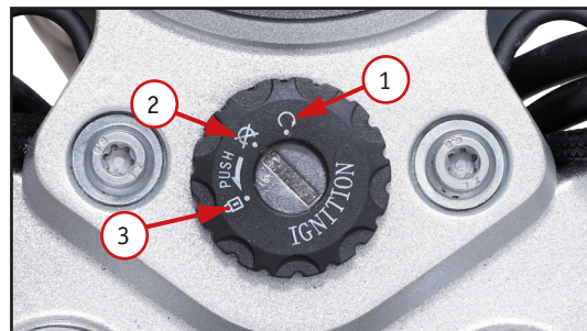
Фото 2.8 Вид замка зажигания: 1 – положение включения питания «☺»; 2 – положение выключения питания «☒»; 3 – положение блокировки рулевой колонки
