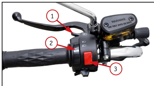
Фото 2.3. Левый комбинированный переключатель: 1 – кнопка включения дальнего света при обгоне; 2 – переключатель дальнего/ближнего света; 3 – кнопка аварийной сигнализации; 4 – переключатель поворотников; 5 – кнопка сигнала (гудок)
