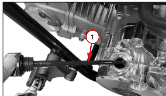
Фото 5.4. Щуп для контроля уровня масла 1
