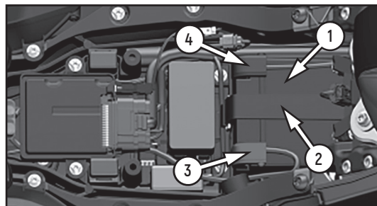
Фото 4.1 Расположение аккумулятора (вариант): 1 – аккумулятор; 2 – ремень; 3 – колпачок клеммы «плюс» (красный провод); 4 – колпачок клеммы «минус» (черный провод)
