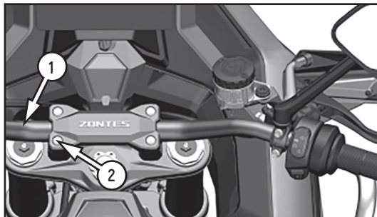
Фото 2.16 Крепление руля (вариант): 1 – руль; 2 – крепежные болты (4 шт.)
