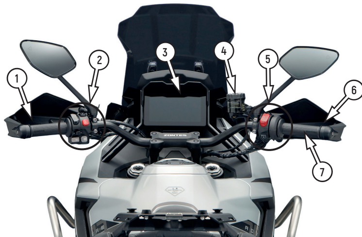
Фото 2.1 Вид руля и органов управления (модель ZT703-F): 1 – рычаг сцепления; 2 – левый блок переключателей; 3 – приборная панель; 4 – бачок для тормозной жидкости передних тормозов; 5 – правый блок переключателей; 6 – ручка переднего тормоза; 7 – ручка газа (акселератора)
