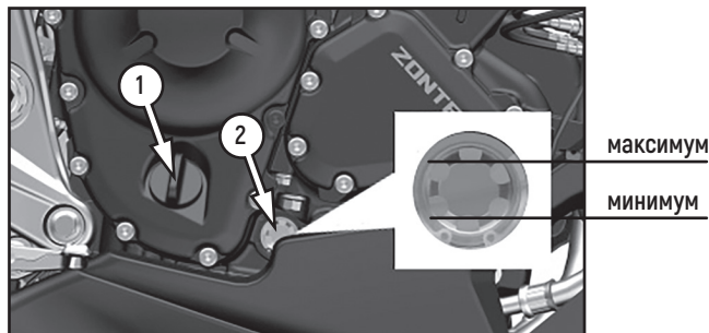
Фото 2.21 Контроль уровня масла в двигателе: 1 – крышка заливной горловины; 2 – смотровое окно
