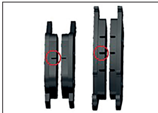
Фото 4.10 Контрольные канавки тормозных колодок
