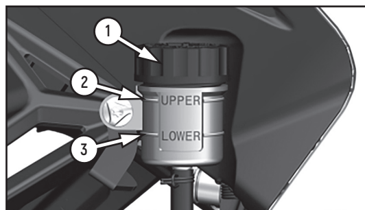
Фото 4.8 Бачки тормозной жидкости переднего и заднего тормозов (вариант): 1 – крышка бачка; 2 – максимальный уровень; 3 – минимальный уровень
