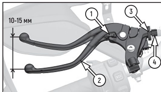
Фото 2.17 Регулировка рычага сцепления (вариант):
