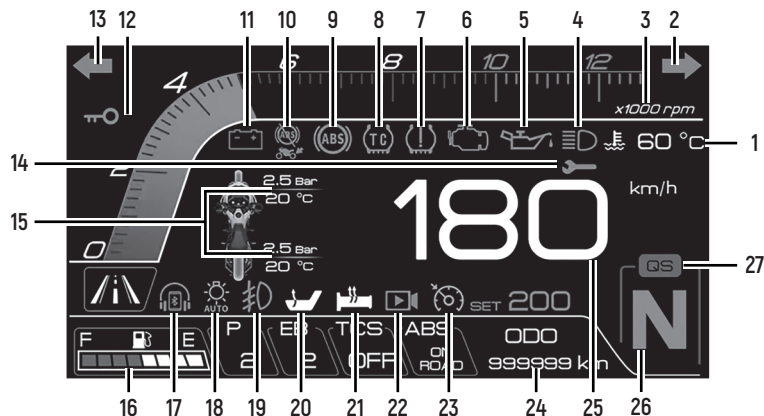
Фото 2.8 Приборная панель (для модели ZT703-F): 1 - индикатор температуры охлаждающей жидкости; 2 - указатель поворота направо; 3 - тахометр "x1000об/мин"; 4 – индикатор дальнего света; 5 - индикатор низкого давления моторного масла; 6 – индикатор неисправности двигателя; 7 – индикатор давления в шинах; 8 - индикатор системы курсовой устойчивости (TCS ); 9 - индикатор системы ABS; 10 – задний индикатор отключения ABS; 11 – индикатор низкого напряжения батареи; 12 – индикатор идентификации ключа; 13 - указатель поворота налево; 14 – индикатор необходимости проведения ТО; 15 – индикация о низком давлении в шинах и температуре; 16 – указатель уровня топлива; 17 – индикатор соединения по Bluetooth; 18 – индикатор автоматического света; 19 – индикатор противотуманных фар; 20 – индикатор обогрева сиденья; 21 – индикатор обогрева ручки; 22 – индикатор работы видео обзора; 23 – индикатор работы круиз контроля; 24 – указатель пройденного расстояния; 25 – указатель текущей скорости; 26 – указатель текущей передачи; 27 – индикатор переключения передач. Для моделей 703-R и 703- RR на панели отображается угол наклона мотоцикла: по середине - в реальном времени; по бокам (лево, право) - максимальные достигнутые углы за поездку. Так же, можно посмотреть отображение времени проезда круга.
