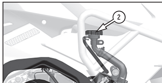
Фото 2.20 Долив охлаждающей жидкости (вариант): 1 – крышка расширительного бачка; 2 – крышка радиатора; «H» – метка максимального уровня; «L» – метка минимального уровня
