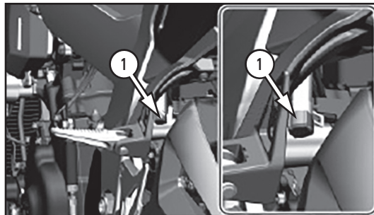
Фото 4.3.1 Расположение трубки слива масла из отсека воздушного фильтра (вариант)
