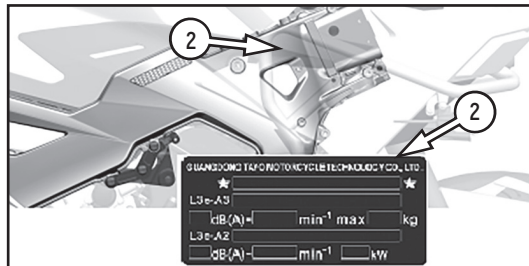
Фото 1.1 Идентификационный номер транспортного средства 1; табличка с VIN номером, датой выпуска и номерами 2
