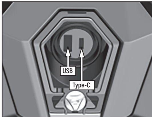
Фото 2.7 Порт зарядки Type-C расположен под крышкой и используется только для зарядки АКБ
