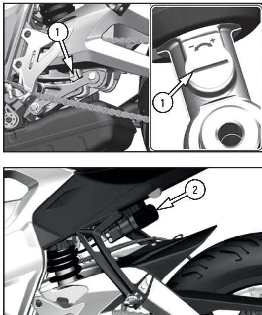
Фото 2.23 Регулировка заднего амортизатора (вариант): 1 - регулировка демпфирования отбоя; 2 - регулировка демпфирования сжатия
