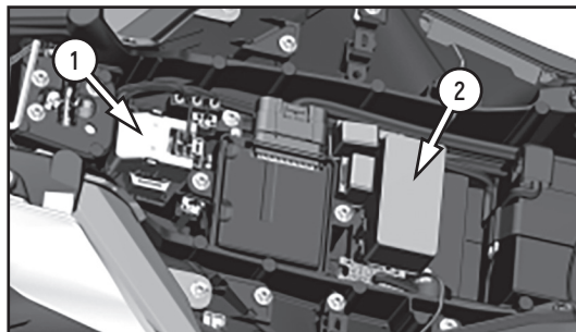
Фото 4.2.1 Размещение предохранителей (вариант): 1 - пусковое реле; 2 – блок предохранителей
