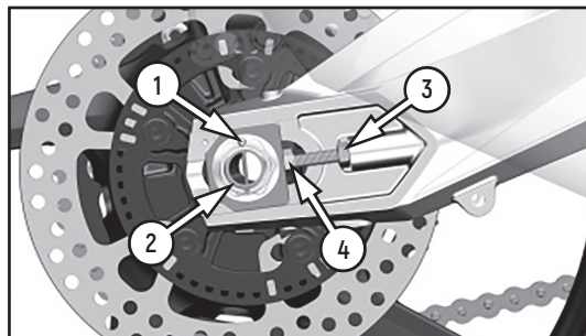
Фото 4.9 Регулировка натяжения цепи (вариант): 1 – шплинт; 2 – гайка оси; 3 – стопорная гайка; 4 – регулировочный болт
