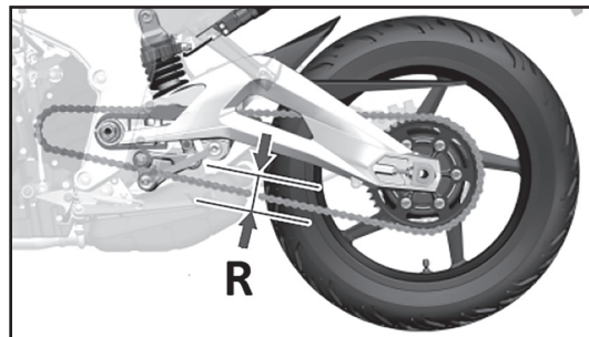
Рисунок 3. Проверка провисания цепи
