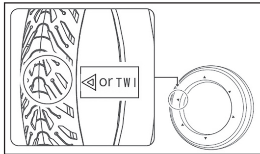
Фото 2.24 Расположение метки износа шины
