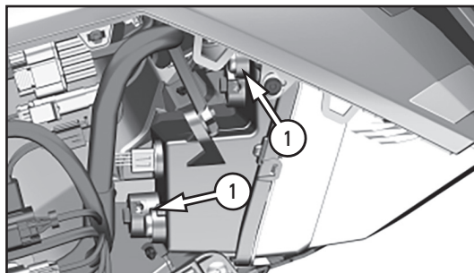
Фото 4.11 Регулировка положения передних фар (модель ZT703-F): 1 – места регулировки
