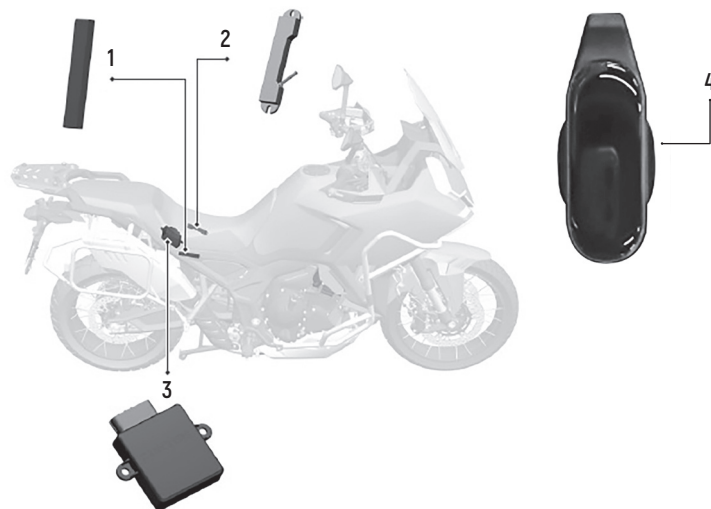
Фото 2.6 Система бесключевого доступа: 1 – приемо-передающая антенна; 2 – индуктивная антенна; 3 – блок управления РЧЕ; 4 – активный ключ
