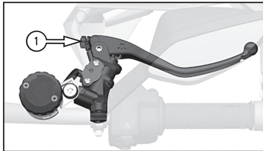
Фото 2.18 Регулировка рычага переднего тормоза (вариант): 1 – болт регулировки
