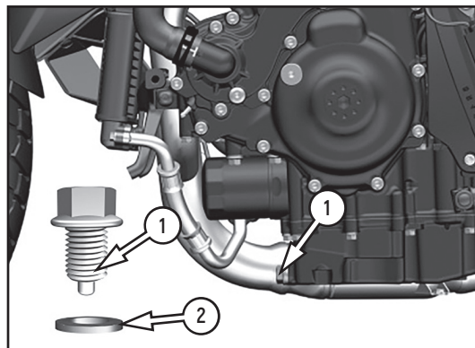
Фото 4.6 Слив моторного масла: 1 – сливной болт; 2 – шайба
