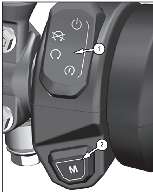
Фото 2.5 Правый блок переключателей: 1 – кнопка включения/отключения двигателя; 2 – кнопка включения режимов работы
