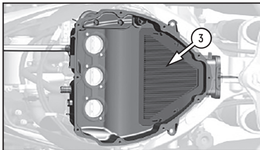
Фото 4.3 Снятие воздушного фильтра (вариант): 1 – винт крепления (10 штук); 2 – картридж воздушного фильтра; 3 – картридж воздушного фильтрующего элемента
