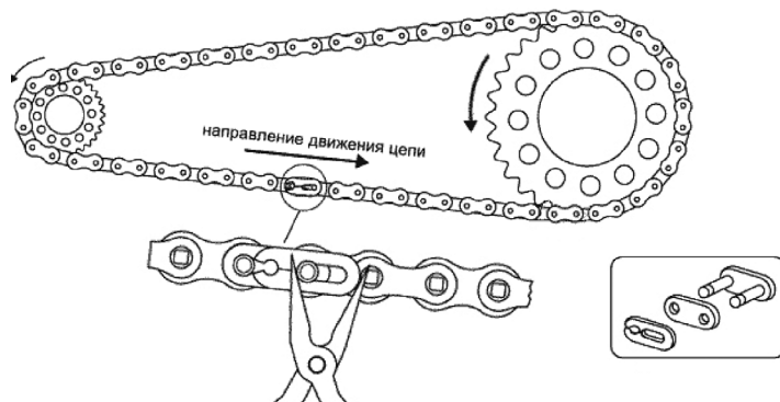
Рисунок 5.26. Установка элементов замка цепи
