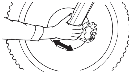
Рисунок 5.27. Проверка рулевой колонки
