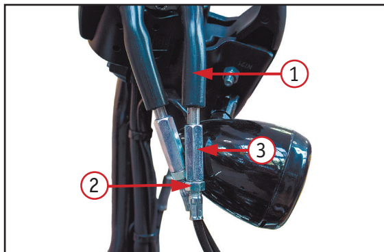
Фото 3. Регулировка троса газа: 1 – защитный колпачок; 2 – стопорная гайка; 3 – регулировочная гайка
