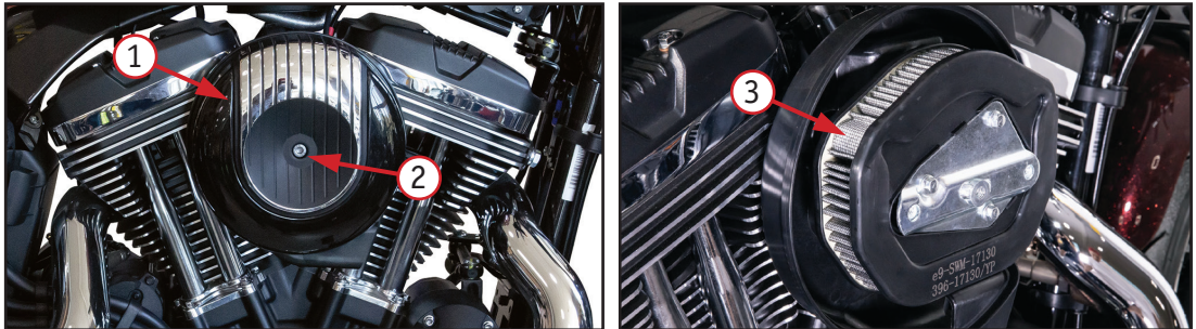
Фото 5.1 Воздушный фильтр: 1 – крышка, 2 – винт крепления; 3 - фильтр
