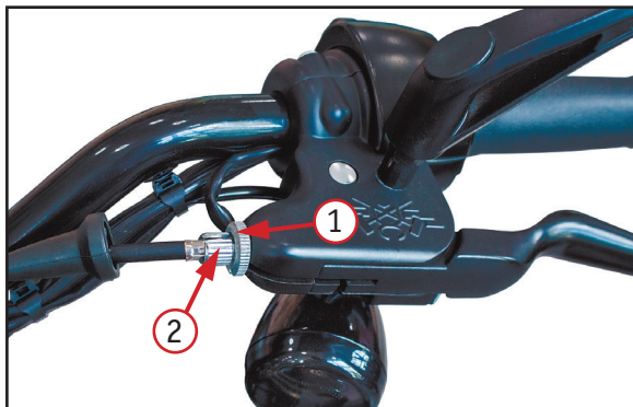
Фото 2.11. Регулировка сцепления: 1 – стопорная гайка; 2 – регулировочный винт
