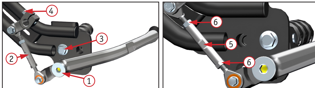
Фото 3.2 Регулировка рычага переключения передач: 1 – болт крепления оси рычага; 2 – тяга рычага переключения передач с регулировочными винтами; 3 – болт крепления подножки водителя; 4 – шлицевое коромысло; 5 – тяга рычага переключения передач; 6 – регулировочные винты
