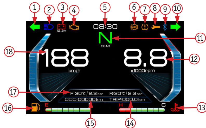
Фото 2.7. Приборная панель: 1 – индикатор левого поворота; 2 – индикатор дальнего света; 3 – индикатор напряжения аккумулятора; 4 – индикатор неисправности двигателя; 5 – часы; 6 – индикатор системы ABS; 7 – индикатор низкого давления в шинах; 8 – индикатор T0; 9 – индикатор Bluetooth-подключения; 10 – индикатор правого поворота; 11 – текущая передача; 12 – тахометр; 13 – шкала температуры охлаждающей жидкости; 14 – текущий километраж; 15 – общий километраж; 16 – шкала уровня топлива; 17 – температура воздуха/давление в шинах; 18 – спидометр
