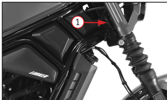
Фото 1.2 Идентификационный код транспортного средства (VIN) – 1 нанесен на правой стороне мотоцикла на раме
