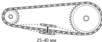
Рисунок 4. Натяжение цепи
