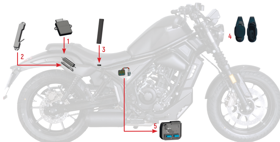
Фото 2.6.1 Компоненты системы бесключевого доступа: 1 – основной модуль РКЕ (иммобилайзер); 2 – индуктивная антенна без питания; 3 – низкочастотная передающая антенна; 4 – беспроводной ключ; 5 – блок порта зарядки с предохранителями
