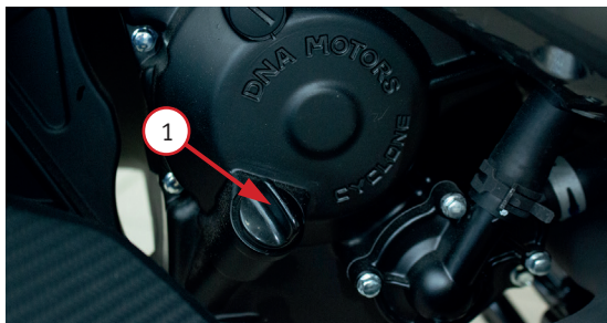
Фото 5.4. Пробка с щупом контроля уровня масла 1
