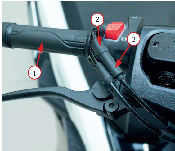
Фото 3. Регулировка троса газа: 1 – ручка газа (акселератора); 2 – стопорная гайка; 3 – регулировочная гайка.
