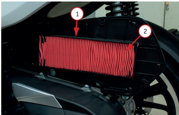
Фото 5.1. Снятие воздушного фильтра: 1 – пластиковый корпус воздушного фильтра; 2 – фильтрующий элемент
