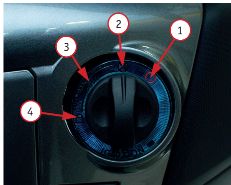
Фото 2.9. Замок зажигания имеет четыре положения: 1 – зажигание включено; 2 – зажигание выключено; 3 – поворот в этом секторе против часовой стрелки откроет крышку доступа к бензобаку; 4 – при нажатии на переключатель и повороте против часовой стрелки в положение происходит блокировка руля.
