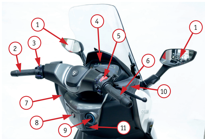
Фото 2.1. Вид руля и органов управления скутера: 1 – зеркало заднего вида; 2 – левая рулевая рукоятка; 3 – левый комбинированный переключатель; 4 – приборная панель; 5 – правый комбинированный переключатель; 6 – рукоятка газа (акселератор); 7 – крышка отсека доступа к топливному баку; 8 – замок вещевого ящика; 9 – замок зажигания; 10 – отсек для заливки охлаждающей жидкости; 11 – кнопка открытия сиденья
