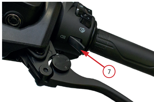
Фото 2.4. Левый комбинированный переключатель: 1 – кнопка подъема ветрового стекла; 2 – кнопка опускания ветрового стекла; 3 – клавиша «MODE» – «SET» (для настройки панели); 4 – переключатель режима фары (дальний / ближний); 5 – клавиша указателей поворотов; 6 – клавиша подачи звукового сигнала; 7 – клавиша включения дальнего света фары при обгоне
