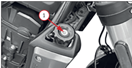
Фото 5.7. Замена охлаждающей жидкости: 1 – крышка радиатора; 2 – крышка бачка; 3 – бачок
