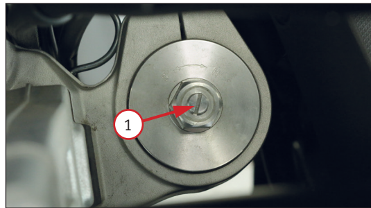
Фото 2.13. Регулировка демпфирования передних и заднего амортизаторов: регулировочный винт 1
