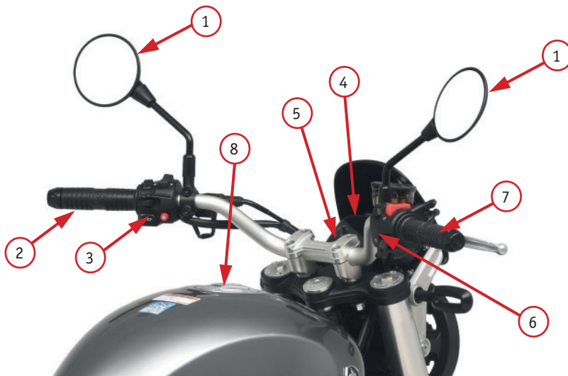
Фото 2.1. Вид руля и органов управления мотоцикла: 1- зеркало заднего вида; 2 - левая рулевая рукоятка; 3 - левый комбинированный переключатель; 4 – приборная панель; 5 - замок зажигания (рядом с панелью); 6 - правый комбинированный переключатель; 7 - рукоятка газа (акселератор); 8 - крышка топливного бака
