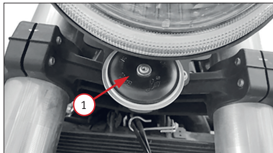
Фото 4.1. 1 - Регулировочный винт электрического звукового сигнала
