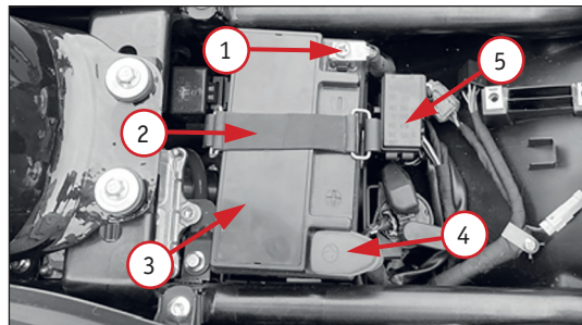
Фото 4. Аккумуляторный отсек: 1 – клемма «минус»; 2 – ремень крепления аккумуляторной батареи; 3 – аккумуляторная батарея (АКБ); 4 – колпачок клеммы «плюс»; 5 – блок предохранителей
