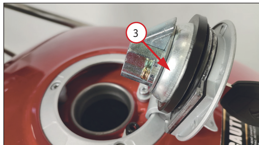
Фото 2.5. Топливный бак: 1 - защитная створка замочной скважины топливного бака; 2 - замочная скважина топливного бака; 3 - крышка топливного бака в открытом положении.
