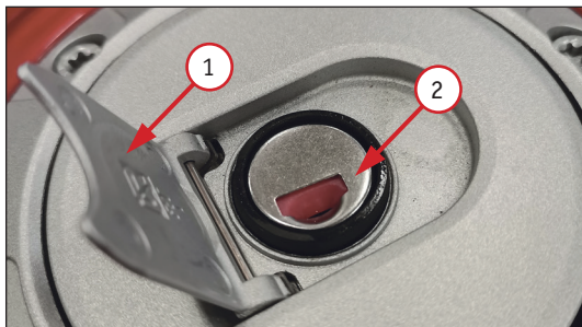
Фото 2.5. Топливный бак: 1 - защитная створка замочной скважины топливного бака; 2 - замочная скважина топливного бака; 3 - крышка топливного бака в открытом положении.
