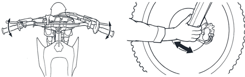
Рисунок 4. Проверка рулевой колонки
