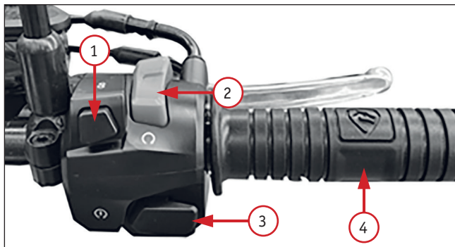
Фото 2.4. Правый комбинированный переключатель: 1 – включатель «S» (функция аналогична кнопке «SET» на левом блоке); 2 - переключатель включения/отключения питания; 3 – кнопка электростартера; 4 – ручка газа (акселератора)
