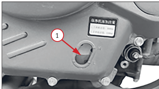
Фото 5.4. Смотровое окно контроля уровня масла 1
