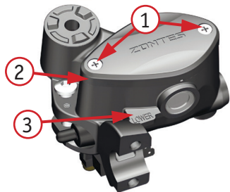
4.8.1. Бачок тормозной жидкости передних тормозов: 1 – винты крепления крышки бачка; 2 – крышка бачка; 3 – уровень «минимум»
