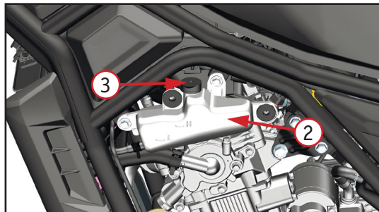
Фото 3.8. Доливание охлаждающей жидкости: 1 – крышка радиатора; 2 – расширительный бачок; 3 – крышка расширительного бачка
