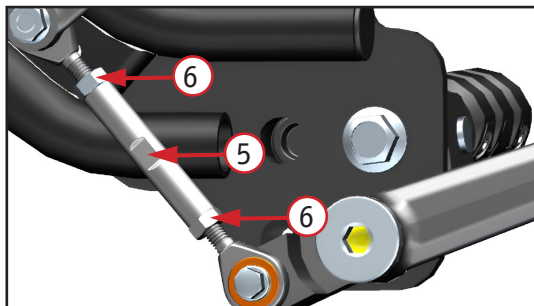
Фото 3.2 Регулировка рычага переключения передач: 1 – болт крепления оси рычага; 2 – тяга рычага переключения передач с регулировочными винтами; 3 – болт крепления подножки водителя; 4 – шлицевое коромысло; 5 – тяга рычага переключения передач; 6 – регулировочные винты
