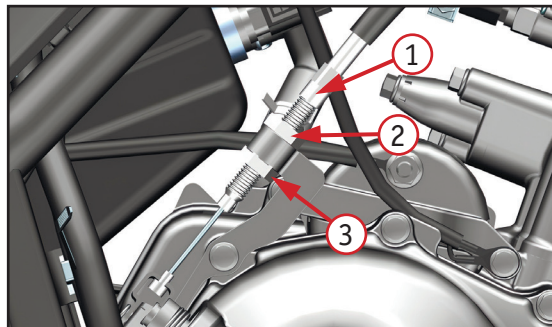
Фото 3.5. Регулировка сцепления на двигателе:
