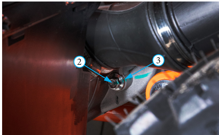
Фото 5.4.2 Залив масла в редуктор (левая сторона): болт 2 смотрового окна уровня масла; 3 – уплотнительная шайба
