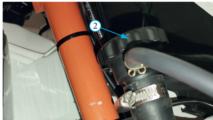
Фото 5.24. Крышка радиатора -2
