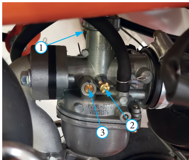
Фото 5.5 Регулировка карбюратора:
