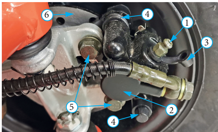
Фото 5.12. Тормозной узел:
