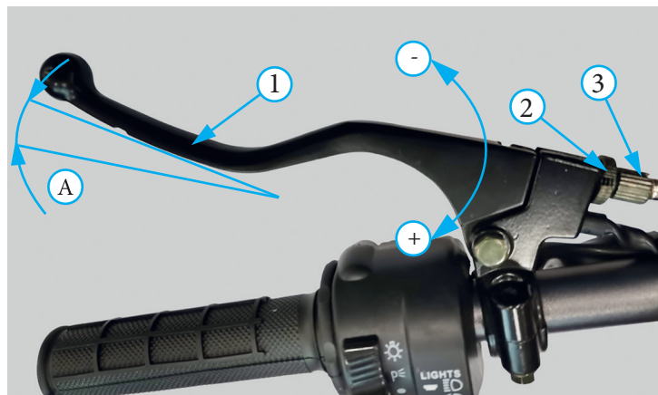
Фото 5.6. Регулировка свободного хода рычага сцепления
