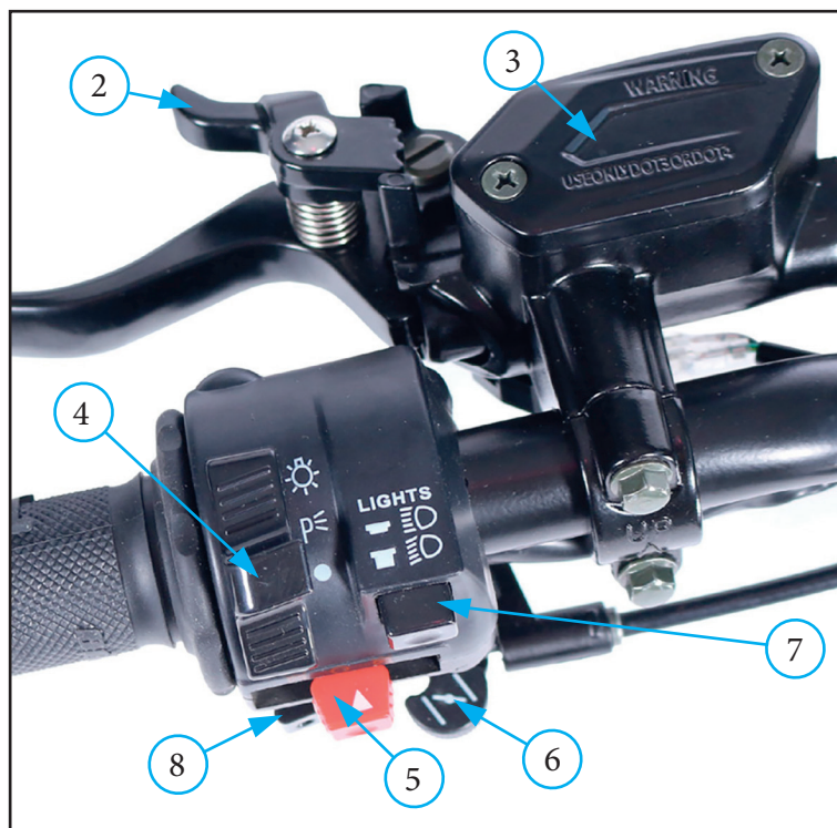
Фото 2.6. Переключатели левого блока квадрицикла (вариант): 1 – рычаг заднего тормоза (рычаг сцепления для моделей с механической трансмиссией); 2 – фиксатор парковочного тормоза; 3 – бачок заднего тормоза; 4 – клавиша включения/выключения света; 5 – кнопка электростартера (вкл./выкл. двигателя); 6 – рычаг обогащения смеси; 7 – кнопка переключения режимов фары; 8 – кнопка сигнала (опция)
