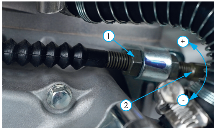
Фото 5.7. Регулировка сцепления на двигателе
