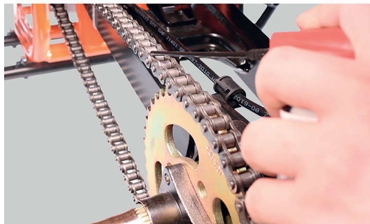
Фото 5.17. Очистка и смазка цепи
