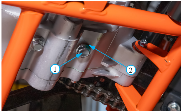
Фото 5.4.1 Слив масла из редуктора: 1 – болт сливного отверстия; 2 – уплотнительная шайба
