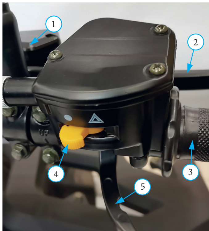
Фото 2.5.1 Переключатели правого рулевого блока квадрицикла (вариант): 1 – бачок переднего тормоза; 2 – рычаг переднего тормоза; 3 – правая ручка; 4 – включатель аварийных сигналов; 5 – рычаг акселератора
