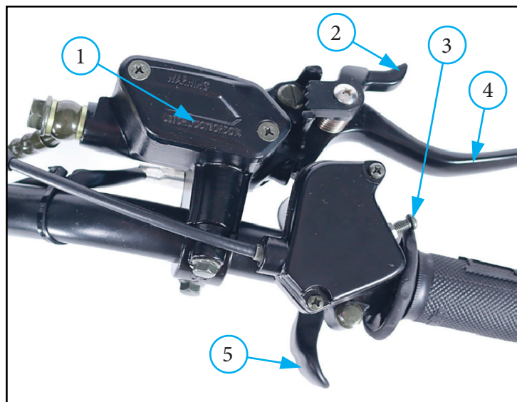
Фото 2.5. Переключатели правого рулевого блока квадрицикла (вариант): 1 - бачок переднего тормоза; 2 - фиксатор парковочного тормоза; 3 - регулятор ограничения акселератора; 4 - рычаг переднего тормоза; 5 - рычаг акселератора
