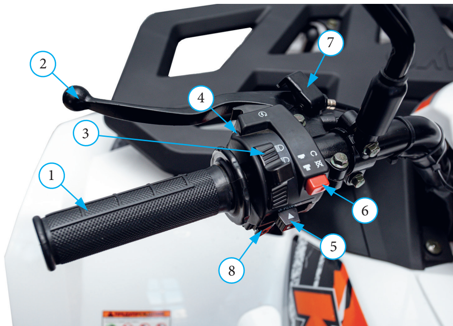
Фото 2.8. Переключатели левого блока квадрицикла (вариант): 1 – левая ручка; 2 – стояночный тормоз; 3 – переключатель фары (выключено/ближний/ дальний); 4 – кнопка электростартера; 5 – включатель указателей поворота; 6 – кнопка включения питания; 7 – фиксатор стояночного тормоза; 8 – кнопка звукового сигнала
