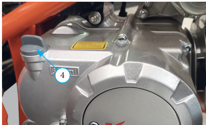
Фото 5.2. Варианты исполнения смотрового окна и крышки горловины двигателей: 1 - смотровое окно с указателями уровня (максимум - «2» и минимум - «3»); 4 - крышка маслозаливной горловины
