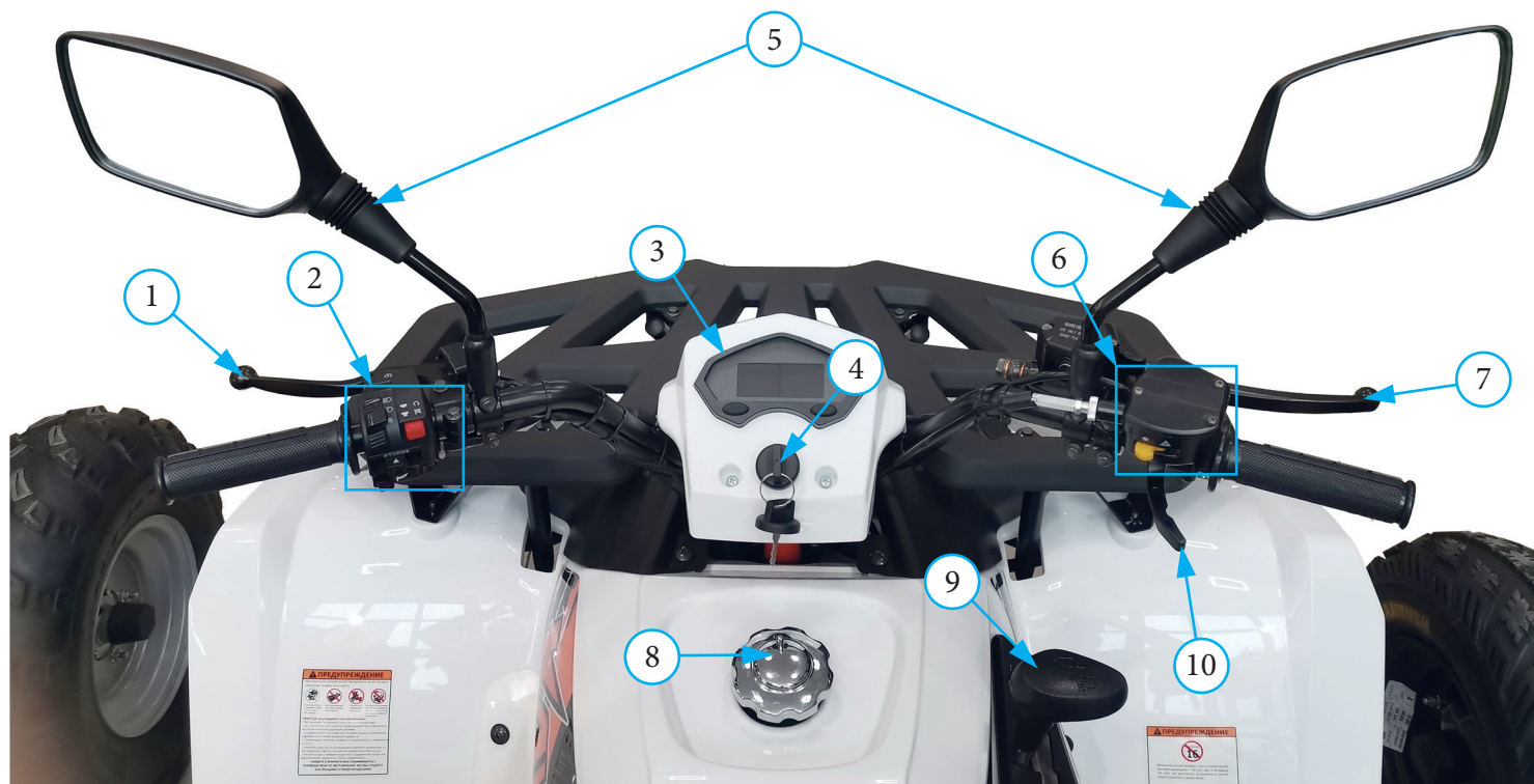
Фото 2.2.1 Приборы и органы управления квадрицикла (вариант): 1 – рычаг сцепления; 2 – левый рулевой блок; 3 – приборная панель; 4 – замок с ключом зажигания; 5 – зеркала заднего вида; 6 – правый рулевой блок; 7 – ручка переднего тормоза; 8 – крышка топливного бака; 9 – рычаг переключения передач; 10 – рычаг акселератора
