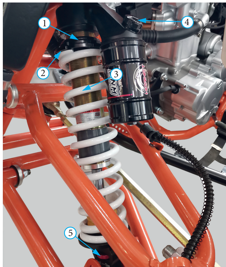
Фото 5.21. Регулировка преднатяга пружины переднего амортизатора и системы демпфирования: 1 – гайка контровочная; 2 – гайка регулировочная; 3 – пружина; 4 – гайка регулировки сжатия; 5 – гайка регулировки отбоя
