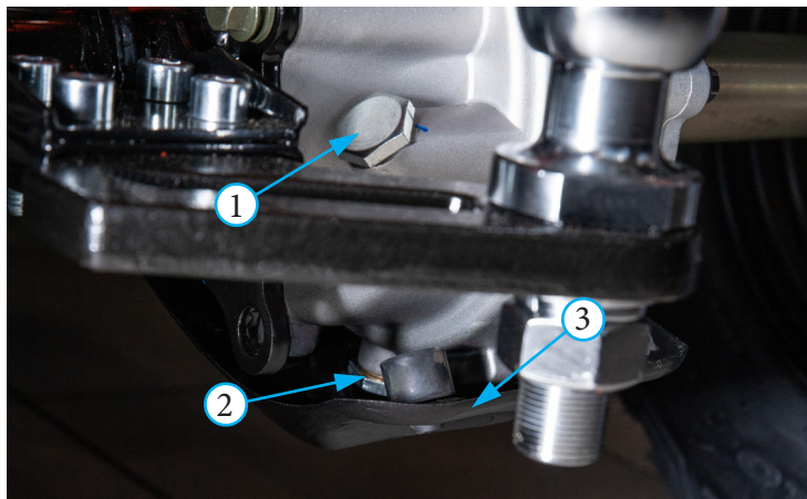
Фото 5.4.3 Замена масла в редукторе заднего моста: 1 – болт заливной горловины; 2 – болт сливного отверстия; 3 – защита редуктора
