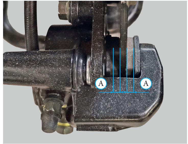
Фото 5.11. Контроль тормозных колодок
