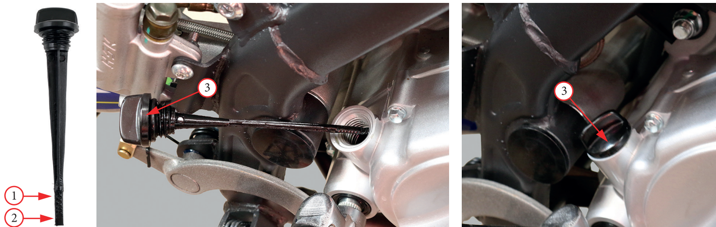
Фото 5.4. Указатель уровня масла в двигателях
