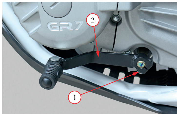
Фото 5.12. Регулировка положения рычага передач
