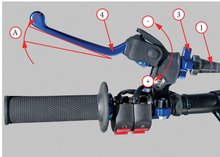
Фото 5.10. Регулировка свободного хода рычага сцепления (варианты исполнения)
