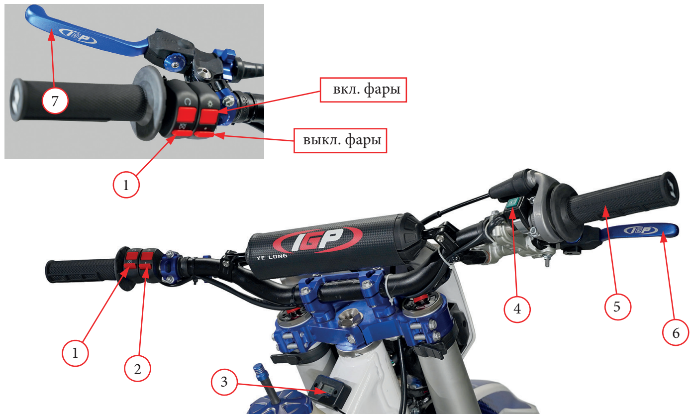
Фото 2.3. Приборы и органы управления спереди мотоцикла: 1 - кнопка выключения двигателя; 2 - кнопка включения/выключения фары; 3 - счетчик моточасов (приборная панель); 4 - кнопка запуска двигателя; 5 - рукоятка акселератора; 6 - рычаг переднего тормоза; 7 - рычаг сцепления
