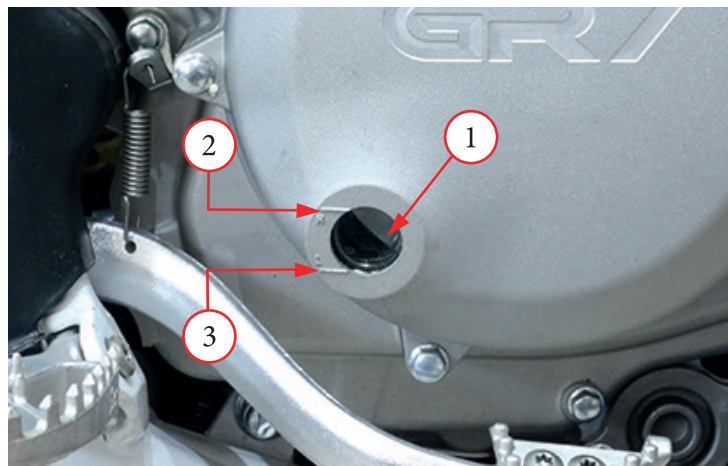
Фото 5.3. Варианты исполнения смотрового окна и крышки горловины двигателей. 1 - смотровое окно с указателями уровня (максимум - «2» и минимум - «3»); 4 – крышка маслозаливной горловины
