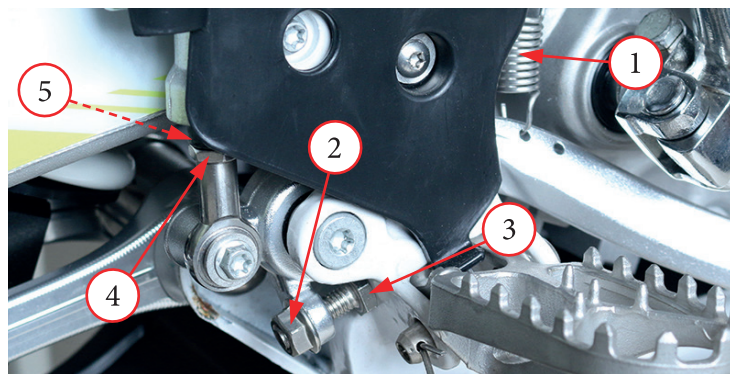
Фото 5.16. Регулировка высоты педали тормоза
