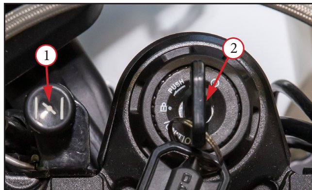
Фото 2.5 Замок зажигания 2 мотоцикла, рычаг обогащения топливной смеси (подсос) 1
