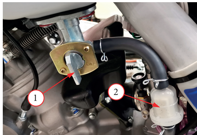
Фото 3.2. Место установки: 1 - топливный кран; 2 - топливный фильтр
