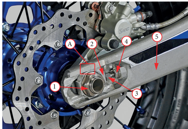
Фото 5.25. Регулировка натяжения цепи
