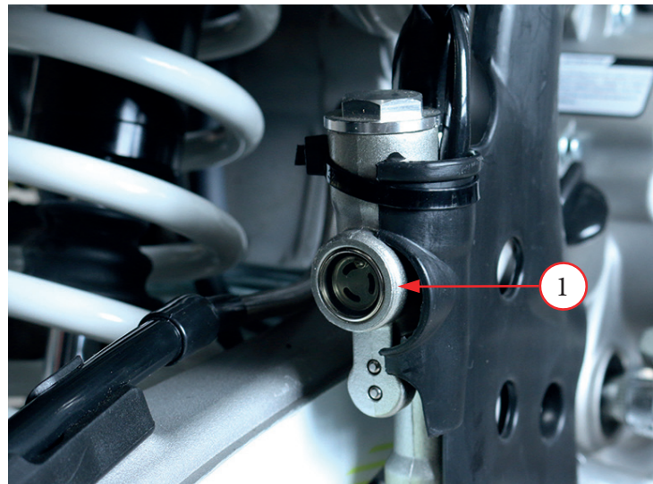
Фото 5.17. Контроль и долив тормозной жидкости
