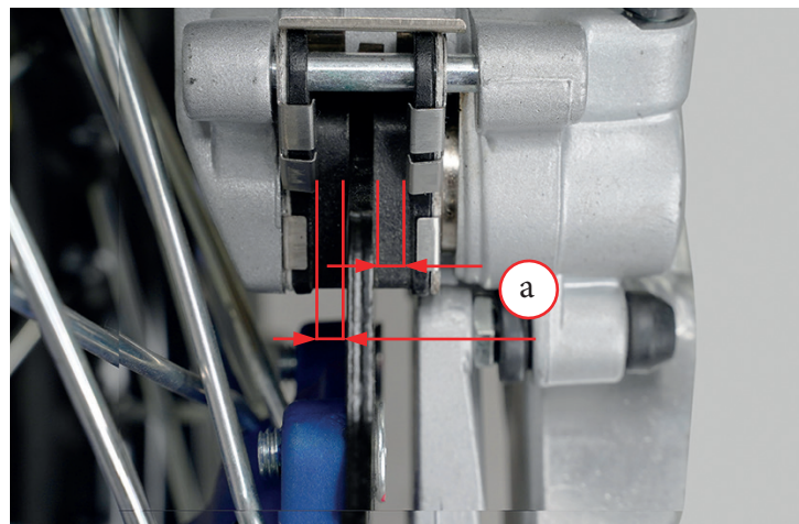
Фото 5.18. Контроль тормозных колодок
