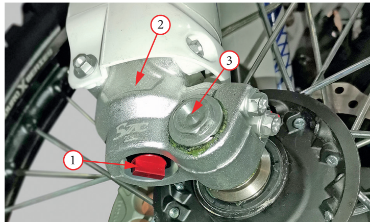
Фото 5.33. Регулировка отбоя передней вилки
