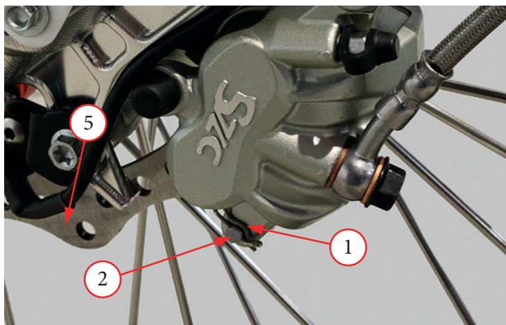
Фото 5.20. Замена передних тормозных колодок
