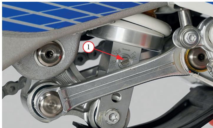
Фото 5.31. Регулировка отбоя задней подвески
