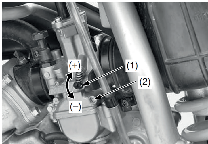
Фото 5.9. Регулировка холостых оборотов
