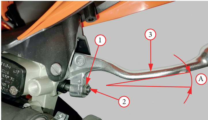
Фото 5.15. Регулировка передних тормозов
