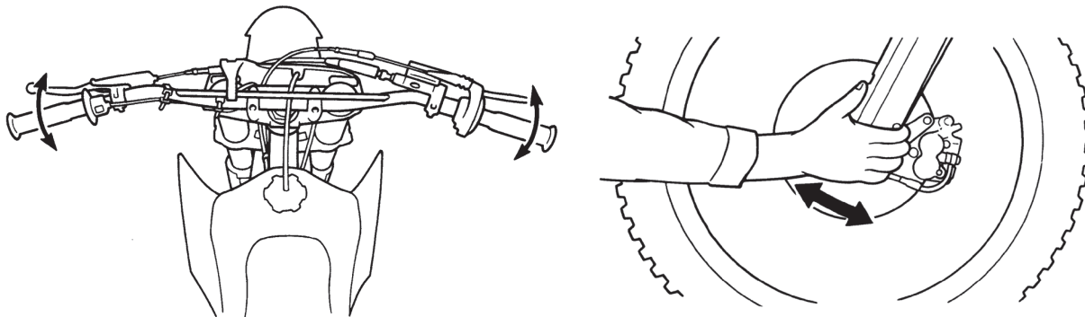
Рисунок 5.27. Проверка рулевой колонки
