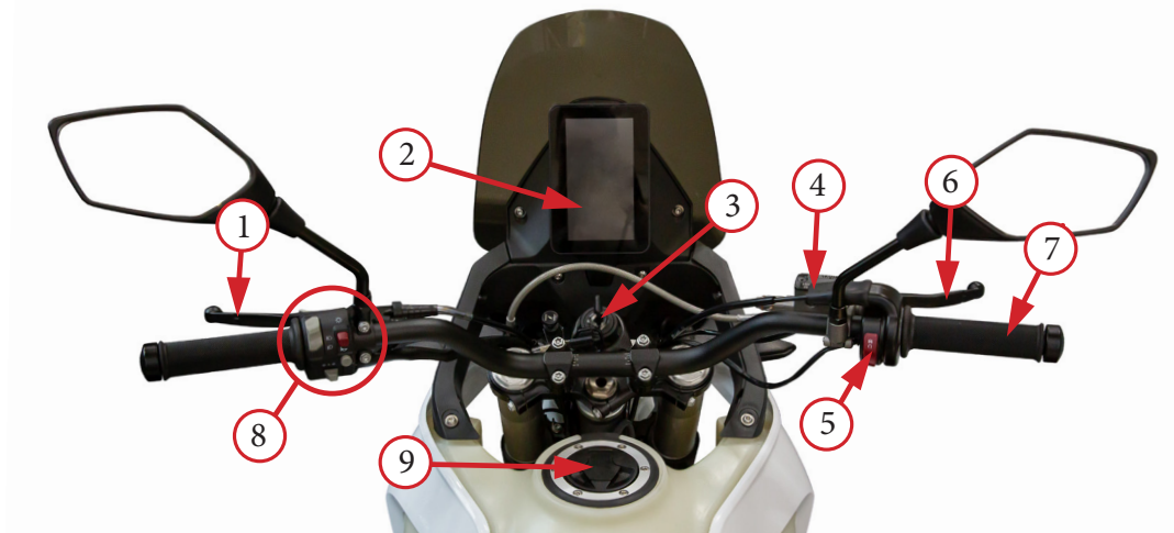
Фото 2.4 Органы управления на примере мотоцикла GR S3 RALLY: 1 – рычаг сцепления; 2 – приборная панель; 3 – замок зажигания; 4 – бачок тормозной жидкости передних тормозов; 5 – кнопка включения/отключения питания двигателя и электростартера; 6 – рычаг переднего тормоза; 7 – ручка акселератора (газа); 8 – левый блок переключателей; 9 – крышка бензобака; 10 – кнопка мигания дальним светом; 11 – кнопка включения света фар; 12 – кнопка переключения режима фары (дальний/ближний свет); 13 – переключатель указания поворотов; 14 – кнопка звукового сигнала
