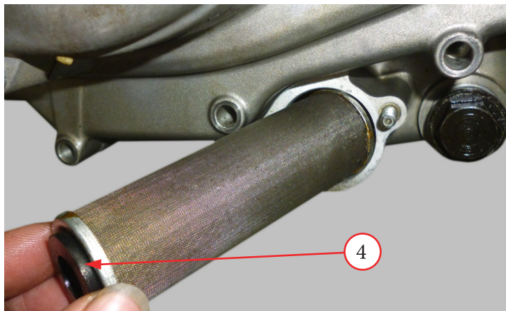
Фото 5.5.1. Замена моторного масла в двигателях с масляным фильтром
