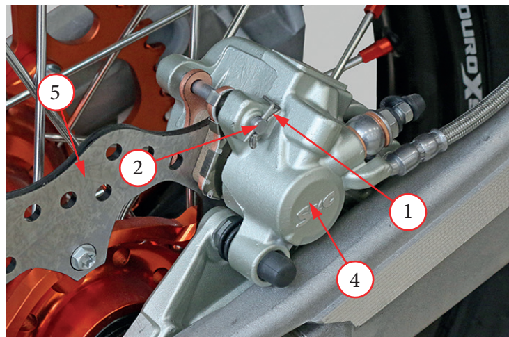
Фото 5.21. Замена задних тормозных колодок
