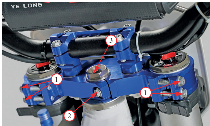
Фото 5.28. Регулировка подшипников рулевой колонки
