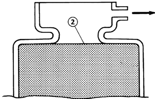
Фото 5.6. Контроль уровня охлаждающей жидкости
