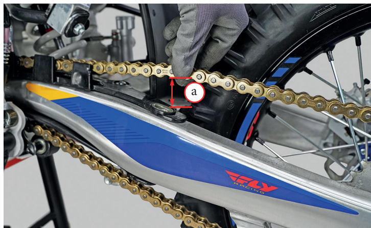
Фото 5.22. Замер провисания цепи
