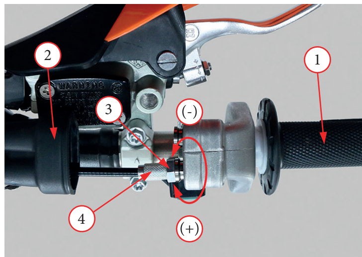
Фото 5.8. Регулировка свободного хода рукоятки акселератора
