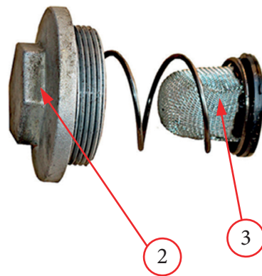
Фото 5.5.3. Замена моторного масла в двигателе с фильтр-сеткой
