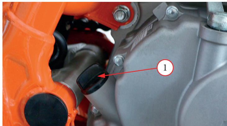
Фото 5.5.3. Замена моторного масла в двигателе с фильтр-сеткой
