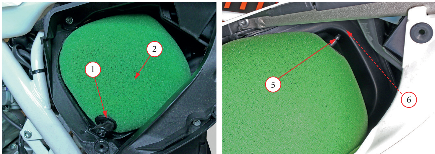
Фото 5.7. Обслуживание воздушного фильтра
