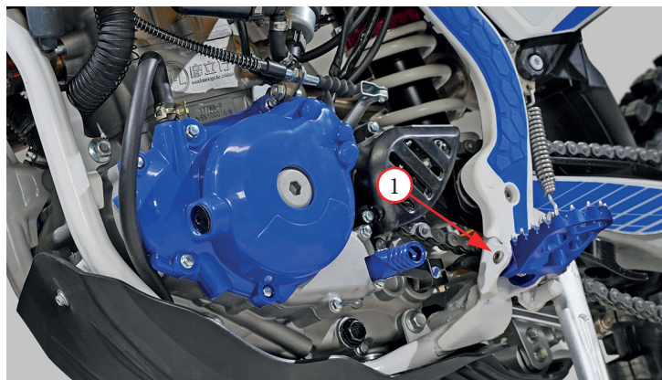
Фото 5.24. Слайдер-успокоитель – 1 (расположен за рамой)
