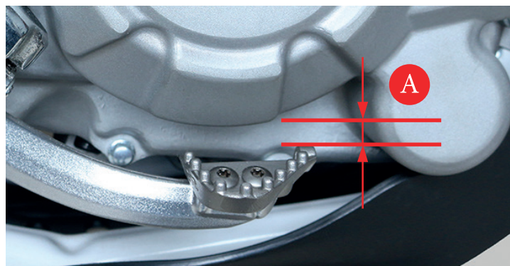
Фото 5.16. Регулировка высоты педали тормоза
