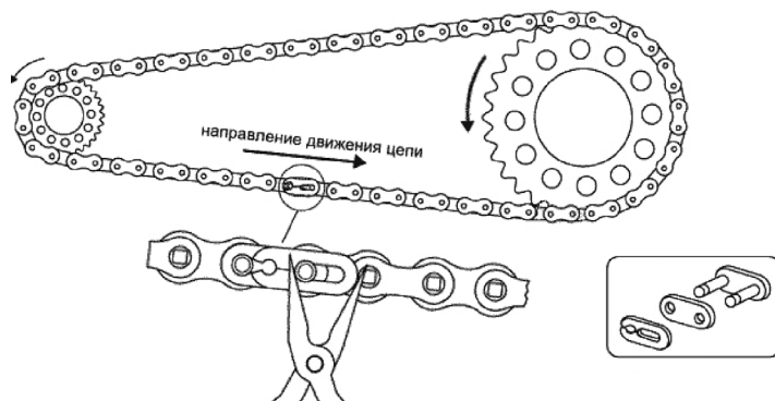
Рисунок 5.26. Установка элементов замка цепи
