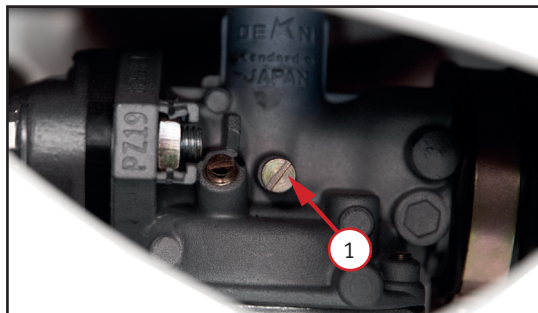
Фото 5.5. Регулировка холостых оборотов: винт регулировки холостых оборотов 1
