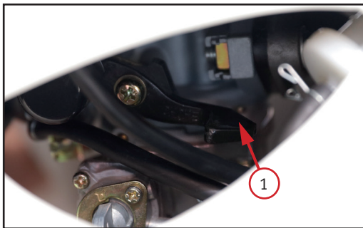
Фото 3.2. Рычаг воздушной заслонки (обогащения топливной смеси) – 1
