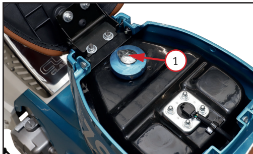
Фото 2.6. Топливный бак: 1 – крышка заливной горловины
