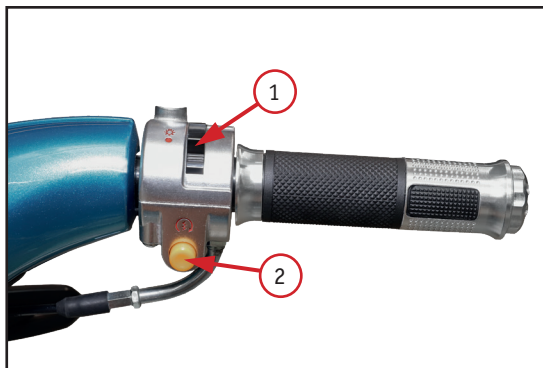
Фото 2.4. Правый комбинированный переключатель: 1 – переключатель освещения; 2 – электростартер
