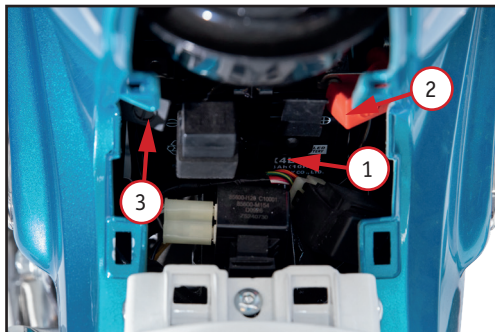
Фото 5.9. Аккумуляторный отсек: 1 — аккумуляторная батарея (АКБ); 2 — клемма «+»; 3 — клемма «-»
