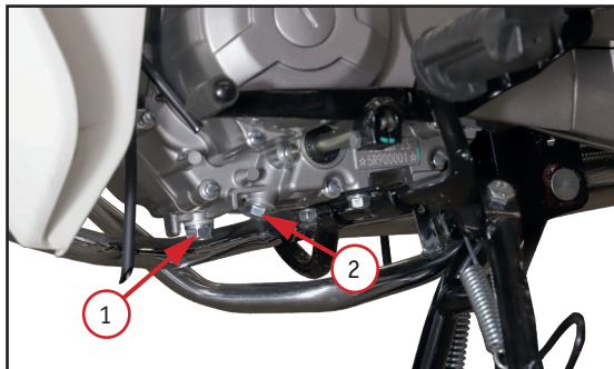
Фото 5.2. Слив масла и чистка фильтра: 1 – сливной болт; 2 – болт крепления сетки грубой очистки
