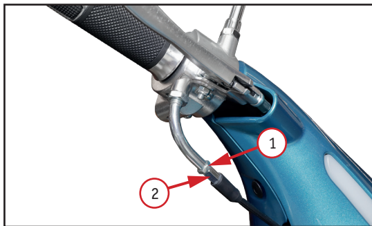
Фото 5.4. Регулировка троса газа: 1 – стопорная гайка; 2 – регулировочная гайка
