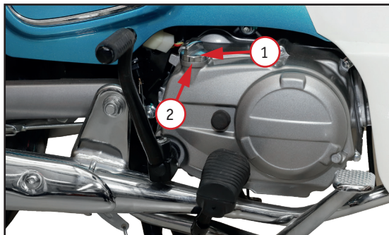
Фото 5.1. Контроль: 1 – щуп контроля уровня масла; 2 – заливная горловина
