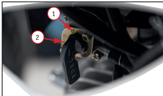
Фото 3.1 Топливный кран: 1 – положение «ОТКРЫТ»; 2 – положение «ЗАКРЫТ»
