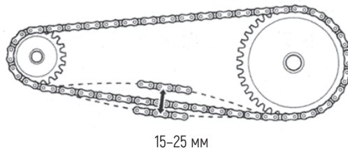
Рисунок 2. Натяжение цепи
