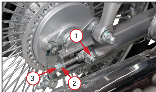
Фото 5.8. Регулировка натяжения цепи: 1 – гайка оси; 2 – регулировочный болт; 3 – стопорная гайка
