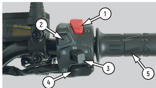
Фото 2.5. Правый комбинированный переключатель: 1 – кнопка включения/отключения питания; 2 – кнопка ABS; 3 - кнопка включения/выключения режимов света; 4 – электростартер; 5 – ручка газа (акселератора)
