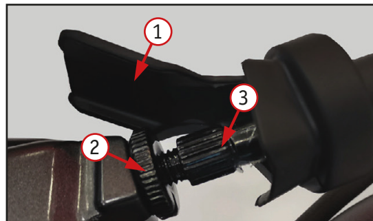
Рисунок 1. Свободный ход рычага сцепления. 1 – резиновый чехол; 2 – стопорная гайка; 3 – регулировочная гайка.
