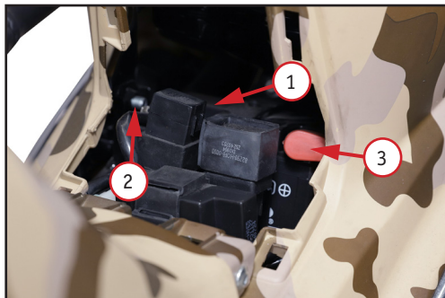
Фото 5.11. Аккумуляторный отсек: 1 — аккумуляторная батарея (АКБ); 2 — клемма «+»; 3 — клемма «-»
