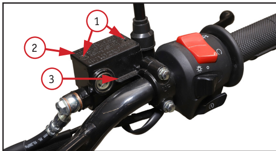
5.8. Бачок тормозной жидкости передних тормозов:
