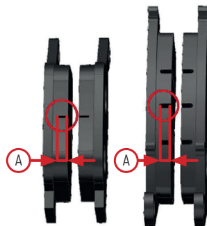
Фото 5.9. Контроль передних тормозных колодок
