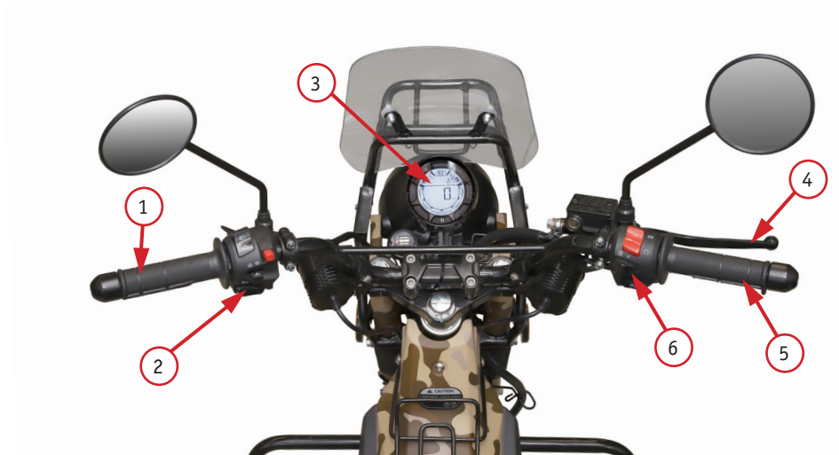
Фото 2.1. Вид руля и органов управления мотоцикла: 1 – левая рулевая рукоятка; 2 – левый комбинированный переключатель; 3 – приборная панель; 4 – правый комбинированный переключатель; 5 – рукоятка газа (акселератор); 6 – ручка переднего тормоза
