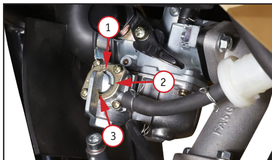
Фото 3.1 Топливный кран: 1 – положение «ОТКРЫТ»; 2 – положение «ЗАКРЫТ»; 3 – положение «РЕЗЕРВ»
