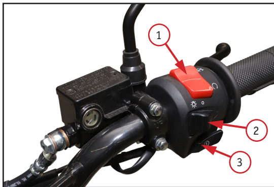
Фото 2.5. Правый комбинированный переключатель: 1 – кнопка включения/отключения питания; 2 – переключатель освещения; 3 – электростартер
