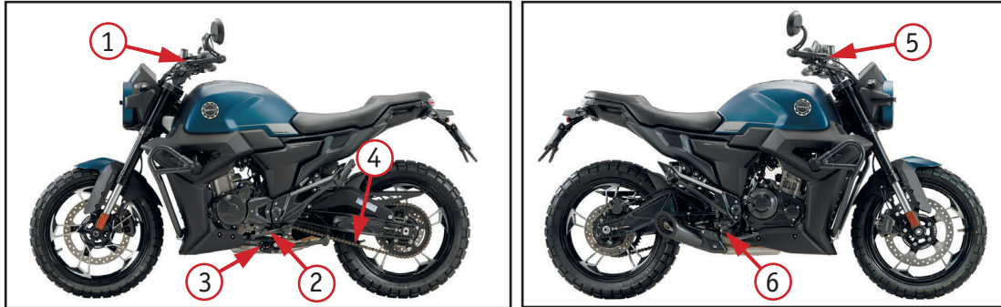
Фото 4.11. Элементы регулярной смазки: 1 – рычаг сцепления; 2 – левая подножка водителя; 3 – боковая подножка с пружиной; 4 – приводная цепь; 5 – рычаг тормоза; 6 – правая подножка водителя
