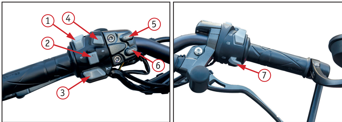
Фото 2.4 Левый комбинированный переключатель: 1 – переключатель режима света фары (дальний свет/ ближний свет); 2 – клавиша указателей поворота; 3 – кнопка звукового сигнала; 4 – кнопка аварийной сигнализации; 5 – кнопка «MOD»; 6 – кнопка «SET»; 7 – кнопка включения дальнего света при обгоне
