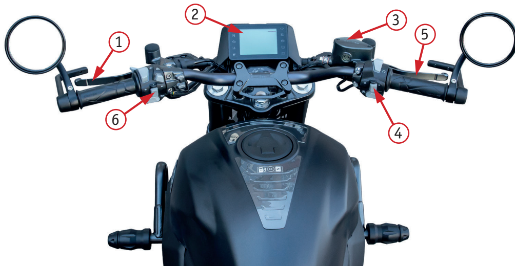
Фото 2.1. Вид руля и органов управления мотоцикла: 1 – рычаг сцепления; 2 – приборная панель; 3 – бачок для тормозной жидкости; 4 – правый комбинированный переключатель; 5 – рычаг переднего тормоза; 6 – левый комбинированный переключатель
