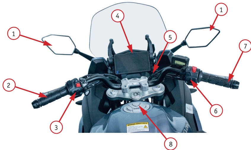
Фото 2.1. Вид руля и органов управления мотоцикла: 1- зеркало заднего вида; 2 - левая рулевая рукоятка; 3 - левый комбинированный переключатель; 4 – приборная панель; 5 - замок зажигания (рядом с панелью); 6 - правый комбинированный переключатель; 7 - рукоятка газа (акселератор); 8 - крышка топливного бака
