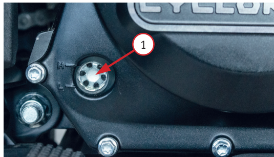
Фото 5. Окно для контроля уровня масла 1
