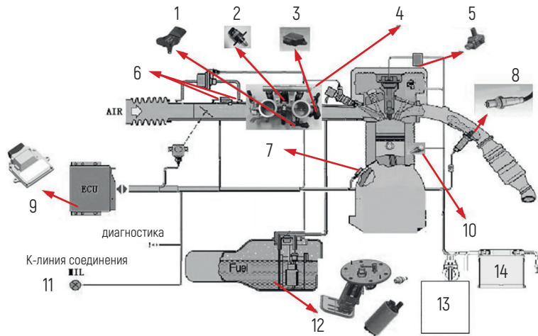
Схема 1. Схема системы EFI: 1 – датчик давления/температуры всасываемого воздуха; 2 – регулятор холостого хода; 3 – датчик положения дроссельной заслонки; 4 – топливный дроссель в сборе; 5 – катушка зажигания; 6 – корпус дроссельной заслонки; 7 – датчик положения коленчатого вала; 8 – датчик кислорода; 9 – электронный блок управления двигателем (ЭБУ); 10 – датчик температуры двигателя; 11 – лампа сигнализации о неисправности; 12 – топливный насос с кронштейном; 13 – насос топливный / клапан регулировки давления / фильтр тонкой очистки; 14 – аккумуляторная батарея (АКБ)
