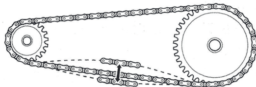
Рисунок 3. Натяжение цепи
