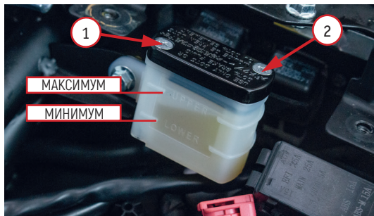
Фото 5.8.1. Бачок тормозной жидкости задних тормозов: 1 – крышка бачка; 2 – винты крепления крышки бачка
