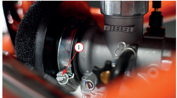
Фото 5.6. Крепление воздушного фильтра
