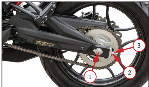
Фото 5.14. Регулировка натяжения цепи: 1 – гайка оси; 2 – регулировочный болт; 3 – стопорная гайка
