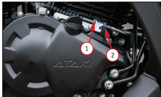
Фото 5.8. Регулировка сцепления на двигателе: 1 – стопорная гайка; 2 – регулятор
