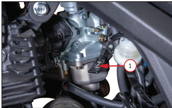
Фото 3.2. Рычаг воздушной заслонки (обогащения топливной смеси) – 1 для моделей CARRERA, CROSSER, WEEK9
