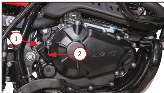
Фото 5.2.2. Контроль уровня масла для моделей CARRERA, CROSSER, WEEK9: 1 – щуп контроля уровня масла; 2 – заливная горловина
