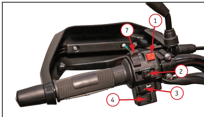
Фото 2.4.2 Левый комбинированный переключатель для модели CROSSER: 1 – переключатель режима света фары (дальний свет/ ближний свет); 2 – клавиша указателей поворота; 3 – кнопка звукового сигнала; 4 – кнопка аварийной сигнализации; 7 – переключатель освещения
