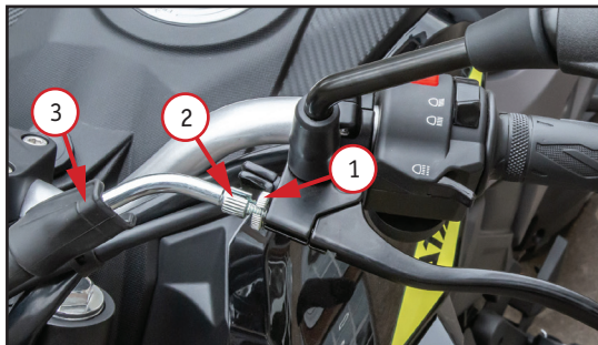
Фото 5.7. Регулировка свободного хода рычага сцепления: 1 – стопорная гайка; 2 – регулятор; 3 – резиновый кожух
