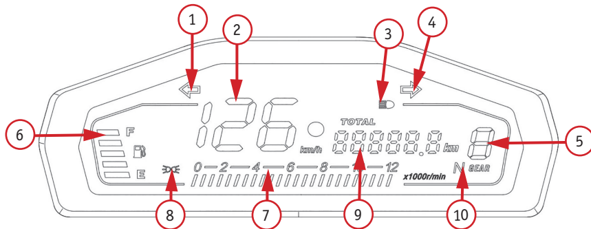
Фото 2.9. Вид приборной панели моделей BATLLO, CARRERA, CROSSER: 1 – индикатор левого поворотника; 2 – скорость; 3 – индикатор дальнего света; 4 – индикатор правого поворотника; 5 – индикатор передачи; 6 – количество топлива; 7 – тахометр; 8 – индикатор габаритных огней; 9 – общий/текущий пробег; 10 – индикатор нейтральной передачи
