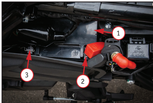
Фото 5.16. Аккумуляторный отсек: 1 – аккумуляторная батарея (АКБ); 2 – клемма «+»; 3 – клемма «-»
