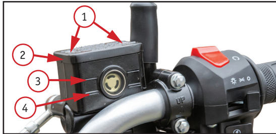
5.11. Бачок тормозной жидкости передних тормозов: 1 – винты крепления крышки бачка; 2 – крышка бачка; 3 – уровень «максимум»; 4 – уровень «минимум»
