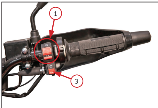
Фото 2.5.2. Правый комбинированный переключатель для модели CROSSER: 1 – переключатель включения/отключения зажигания; 2 – переключатель световых приборов; 3 – кнопка электростартера
