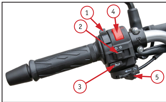
Фото 2.4.1 Левый комбинированный переключатель для моделей BATLLO, CARRERA, WEEK9: 1 – переключатель режима света фары (дальний свет / ближний свет); 2 – клавиша указателей поворота; 3 – кнопка звукового сигнала; 4 – кнопка аварийной сигнализации; 5 –рычаг воздушной заслонки (обоганитель топливной смеси) (только для модели BATLLO); 6 – кнопка включения дальнего света при обгоне
