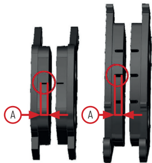
Фото 5.13. Контроль передних и задних тормозных колодок
