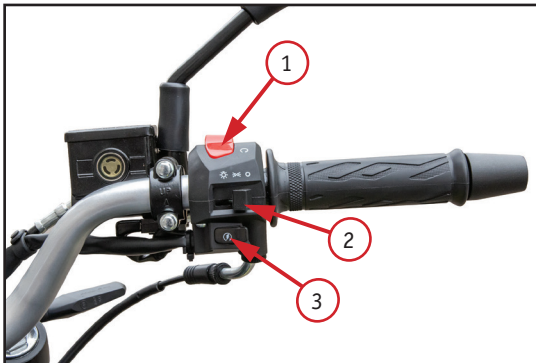
Фото 2.5.1. Правый комбинированный переключатель для моделей BATLLO, CARRERA, WEEK9: 1 – переключатель включения/отключения зажигания; 2 – переключатель освещения; 3 – кнопка электростартера
