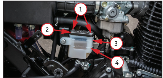
5.12. Бачок тормозной жидкости задних тормозов для моделей BATLLO, CARRERA, CROSSER: 1 – винты крепления крышки бачка; 2 – крышка бачка; 3 – уровень «максимум»; 4 – уровень «минимум»
